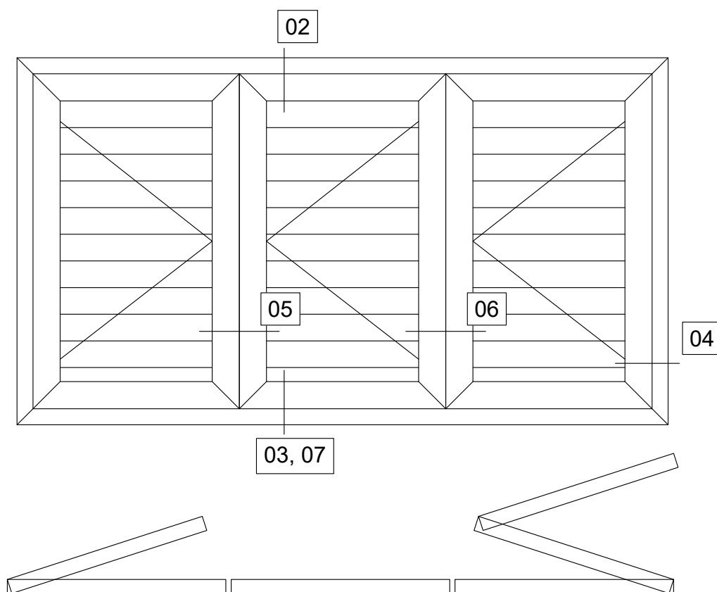
THREE SASH SHUTTER BLINDS FULL FRAME ΤΡΙΦΥΛΛΟ ΠΑΝΤΖΟΥΡΙ ΜΕ ΠΕΡΙΜΕΤΡΙΚΗ ΚΑΣΑ
