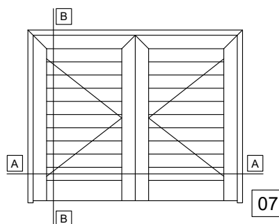
DOUBLE SASH SHUTTER BLINDS WITH KICKPLATE AND WITHOUT THRESHOLD ΔΙΦΥΛΛΟ ΠΑΝΤΖΟΥΡΙ ΜΕ ΤΑΜΠΛΑ ΚΑΙ ΧΩΡΙΣ ΚΑΤΩΚΑΣΙ
