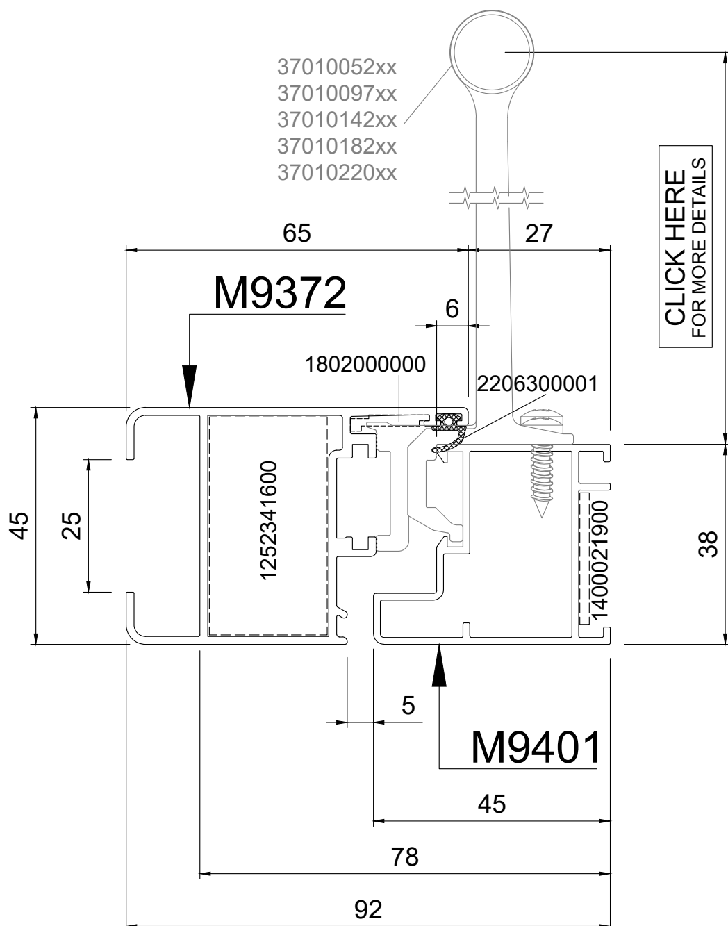
THREE SASH SHUTTER BLINDS FULL FRAME ΤΡΙΦΥΛΛΟ ΠΑΝΤΖΟΥΡΙ ΜΕ ΠΕΡΙΜΕΤΡΙΚΗ ΚΑΣΑ
