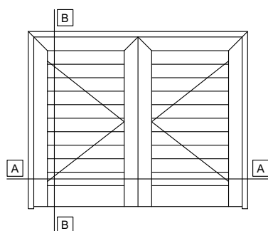
DOUBLE SASH SHUTTER BLINDS WITH KICKPLATE AND WITHOUT THRESHOLD ΔΙΦΥΛΛΟ ΠΑΝΤΖΟΥΡΙ ΜΕ ΤΑΜΠΛΑ ΚΑΙ ΧΩΡΙΣ ΚΑΤΩΚΑΣΙ
