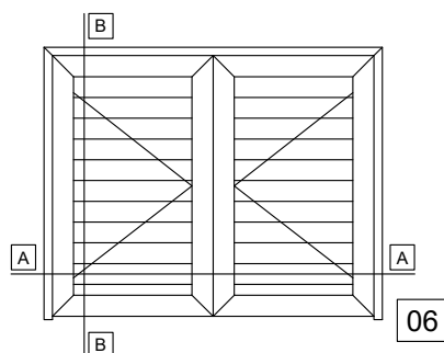
DOUBLE SASH SHUTTER BLINDS WITHOUT THRESHOLD ΔΙΦΥΛΛΟ ΠΑΝΤΖΟΥΡΙ ΧΩΡΙΣ ΚΑΤΩΚΑΣΙ
