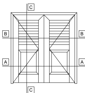
DOUBLE SASH LOUVER / PANEL COMBINATION SHUTTER ΔΙΦΥΛΛΟ ΠΑΝΤΖΟΥΡΙ ΜΕ ΓΑΛΟΝΑΚΙ ΚΑΙ ΤΑΜΠΛΑΔΑΚΙ
