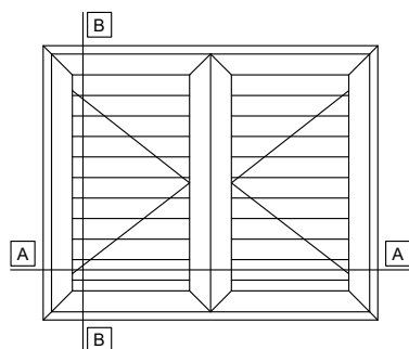
DOUBLE SASH SHUTTER BLINDS FULL FRAME ΔΙΦΥΛΛΟ ΠΑΝΤΖΟΥΡΙ ΜΕ ΠΕΡΙΜΕΤΡΙΚΗ ΚΑΣΑ
