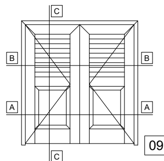
DOUBLE SASH LOUVER / PANEL COMBINATION SHUTTER ΔΙΦΥΛΛΟ ΠΑΝΤΖΟΥΡΙ ΜΕ ΓΑΛΟΝΑΚΙ ΚΑΙ ΤΑΜΠΛΑΔΑΚΙ
