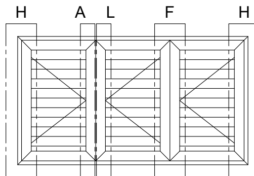
THREE SASH SHUTTER BLINDS FULL FRAME ΤΡΙΦΥΛΛΟ ΠΑΝΤΖΟΥΡΙ ΜΕ ΠΕΡΙΜΕΤΡΙΚΗ ΚΑΣΑ
