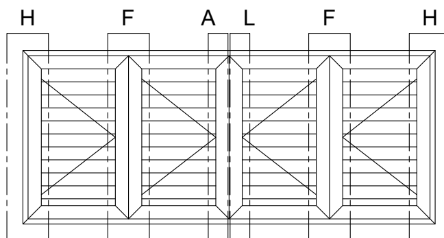
FOUR SASH SHUTTER BLINDS FULL FRAME ΤΕΤΡΑΦΥΛΛΟ ΠΑΝΤΖΟΥΡΙ ΜΕ ΠΕΡΙΜΕΤΡΙΚΗ ΚΑΣΑ
