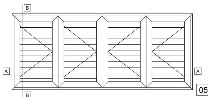
FOUR SASH SHUTTER BLINDS FULL FRAME ΤΕΤΡΑΦΥΛΛΟ ΠΑΝΤΖΟΥΡΙ ΜΕ ΠΕΡΙΜΕΤΡΙΚΗ ΚΑΣΑ
