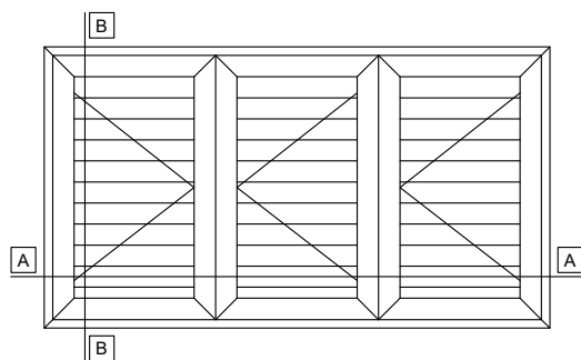
THREE SASH SHUTTER BLINDS FULL FRAME ΤΡΙΦΥΛΛΟ ΠΑΝΤΖΟΥΡΙ ΜΕ ΠΕΡΙΜΕΤΡΙΚΗ ΚΑΣΑ
