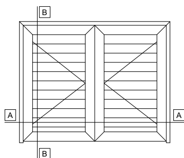
DOUBLE SASH SHUTTER BLINDS WITHOUT THRESHOLD ΔΙΦΥΛΛΟ ΠΑΝΤΖΟΥΡΙ ΧΩΡΙΣ ΚΑΤΩΚΑΣΙ
