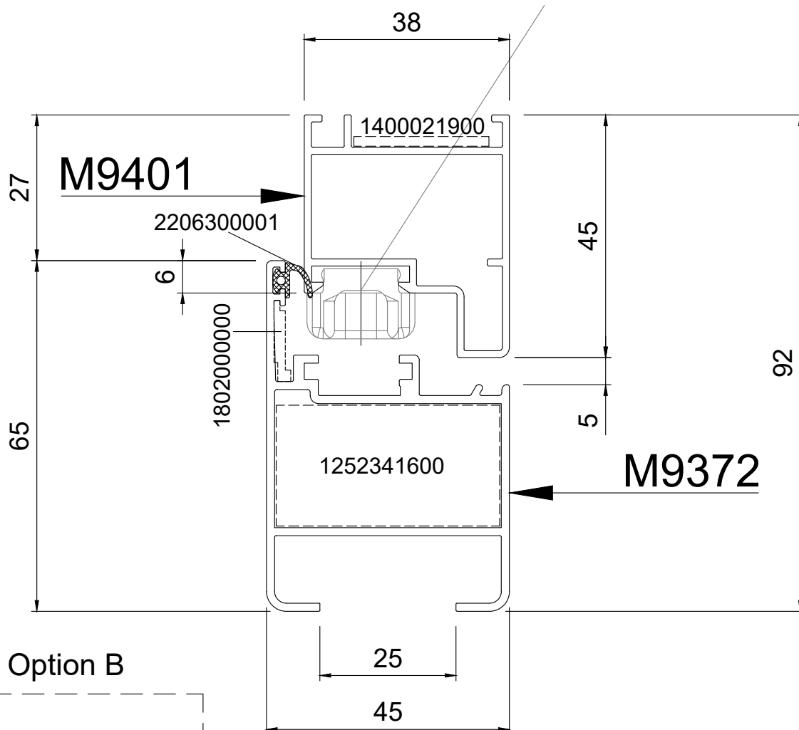
DOUBLE SASH SHUTTER BLINDS FULL FRAME ΔΙΦΥΛΛΟ ΠΑΝΤΖΟΥΡΙ ΜΕ ΠΕΡΙΜΕΤΡΙΚΗ ΚΑΣΑ
