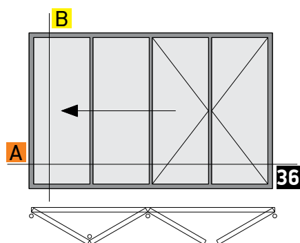
INWARD OPENING, 3+1 4-PANELS FOLDING DOOR ΜΕΣΑ ΑΝΟΙΓΟΜΕΝΗ, 3+1 4-ΦΥΛΛΗ ΦΥΣΟΥΝΑ
