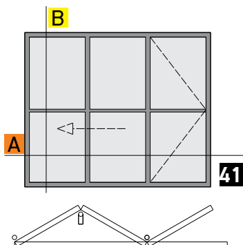
OUTWARD OPENING, 3 PANELS ON ONE SIDE FOLDING DOOR ΕΞΩ ΑΝΟΙΓΟΜΕΝΗ, 3 ΦΥΛΛΗ ΦΥΣΟΥΝΑ ΣΕ ΜΙΑ ΠΛΕΥΡΑ
