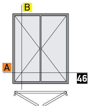
INWARD OPENING, 1+1 2-PANELS DOOR ΜΕΣΑ ΑΝΟΙΓΟΜΕΝΗ, 1+1 2-ΦΥΛΛΗ ΠΟΡΤΑ
