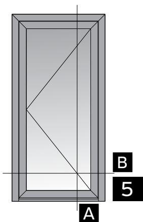
Single sash entrance door opening inward with glass panel with 12mm threshold Μονόφυλλη πόρτα εισόδου ανοιγομένη μέσα με υαλοπίνακα με κατωκάσι 12mm
