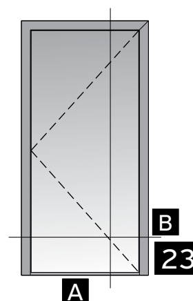
Single sash entrance door opening outward with insulation panel 77 mm Μονόφυλλη πόρτα εισόδου ανοιγόμενη έξω με μονωτικό πάnevλ 77 χιλ.
