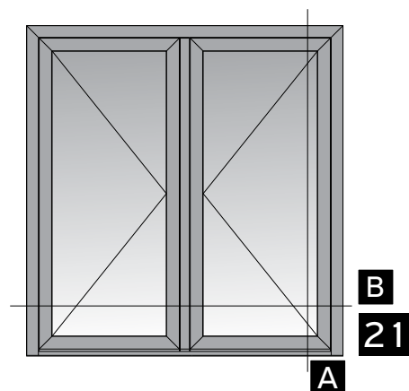
Double sash entrance door opening inward with glass panel with windbarrier Δίφυλλη πόρτα εισόδου ανοιγόμενη μέσα με υαλοπίνακα με ανεμοφράχτη
