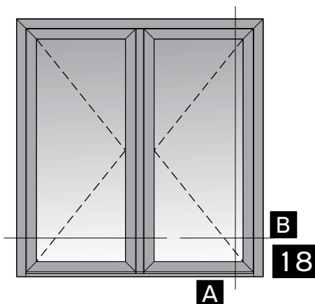
Double leaf entrance door opening outward with narrow reversing mullion Δίφυλλη πόρτα εισόδου ανοιγομένη έξω με μιννόφυλλο
