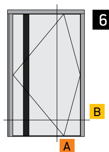
Μονόφυλλη πόρτα εισόδου ανοιγόμενη μέσα με μονωτικό πάνελ 120.5 χιλ. Γαλποπάννα εξωτερικά Single sash entrance door opening inward with insulation panel 120.5 mm Glass pane external
