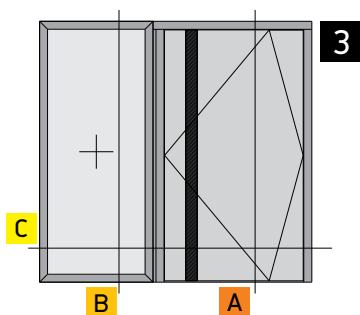
Μονόφυλλη πύλη εισόδου ανοιγόμενη μέσα με μονωτικό πάνελ 115 χιλ. και πλαινό σταθερό με γυαλί Single sash entrance door opening inward with insulation panel 115 mm and fixed side glass panel
