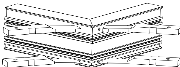
Μαχαίρια για γωνιάστρες Crimp profiles with Knifes
