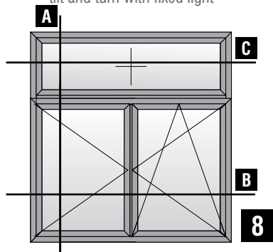
Δίφυλλο ανοιγόμενο - ανακλινόμενο με σταθερό επάνω Double side-hung casement, tilt and turn with fixed light
