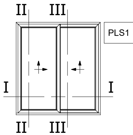
Two Sash Parallel Lift and Slide 45 Degrees Cut Right Sliding Window Δίφυλλο Επάλληλο Δεξιά Ανασυρόμενο με κοπή 45 Μοιρών
