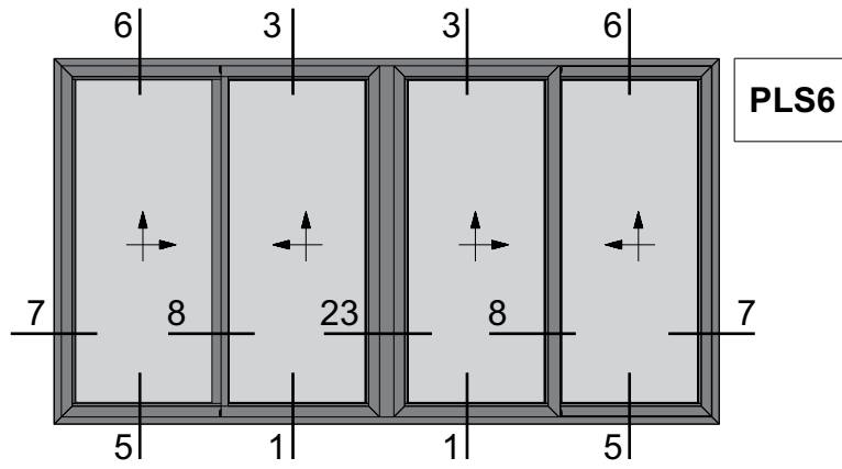
For Sash Parallel Lift and Slide 90 Degrees Cut Right Sliding Window with Meeting Stile Τετράφυλλο Επάλληλο Φιλητό Δεξιιά Ανασυσρόμενο με κοπή 90 Μοιρών
