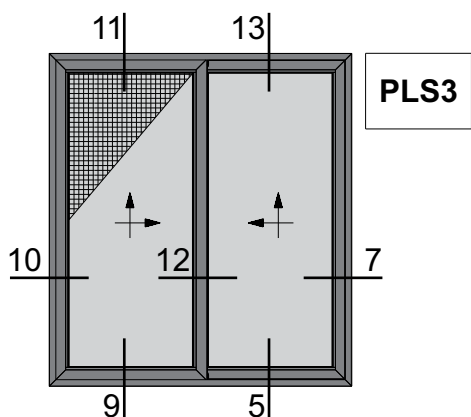
Two Sash Parallel Lift and Slide 45 Degrees Cut Right Sliding Window with Flyscreen Δίφυλλο Επάλληλο Δεξιιά Ανασυσρόμενο με κοπή 45 Μοιρών με Σήτα
