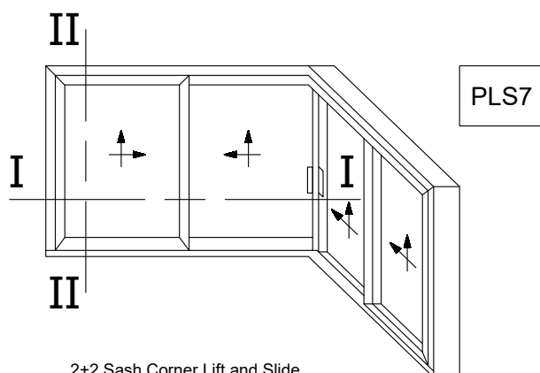
2+2 Sash Corner Lift and Slide 45 Degrees Cut Sliding Window Γωνιακό Επάλληλο Ανασυρόμενο με κοπή 45 Μοιρών
