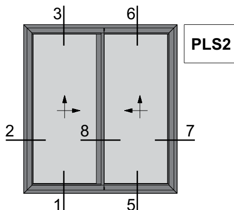
Two Sash Parallel Lift and Slide 90 Degrees Cut Right Sliding Window Δίφυλλο Επάλληλο Δεξιιά Ανασυσρόμενο με κοπή 90 Μοιρών
