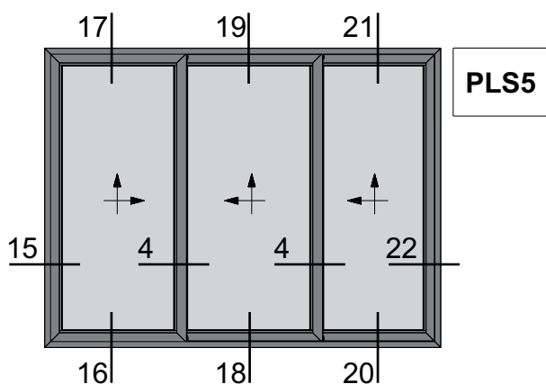
Three Sash Parallel Lift and Slide 45 Degrees Cut Right Sliding Window Τρίφυλλο Επάλληλο Δεξιιά Ανασυσρόμενο με κοπή 45 Μοιρών
