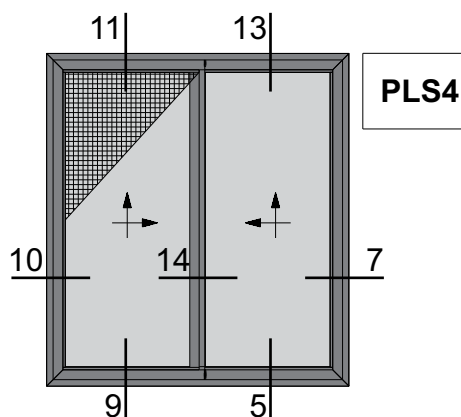
Two Sash Parallel Lift and Slide 90 Degrees Cut Right Sliding Window with Flyscreen Δίφυλλο Επάλληλο Δεξιιά Ανασυσρόμενο με κοπή 90 Μοιρών με Σήτα
