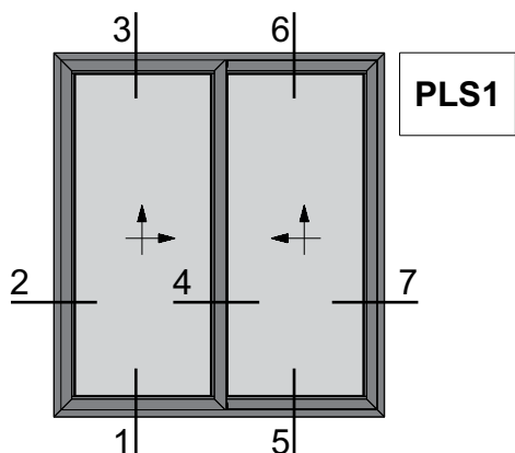
Two Sash Parallel Lift and Slide 45 Degrees Cut Right Sliding Window Δίφυλλο Επάλληλο Δεξιιά Ανασυσρόμενο με κοπή 45 Μοιρών
