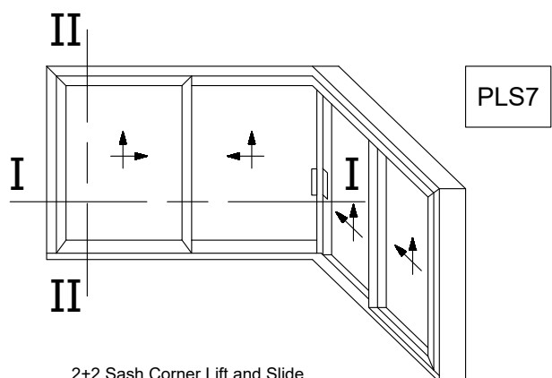
2+2 Sash Corner Lift and Slide 45 Degrees Cut Sliding Window Γωνιακό Επάλληλο Ανασυσρόμενο με κοπή 45 Μοιρών
