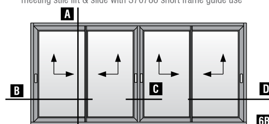
Τετράφυλλο φιλιτό επάλληλο ανασυρόμενο (κοπή 90°) με χρήση χαμηλού οδηγού S70786 Four sash meeting stile parallel lift & slide (90° cutting) with S70786 short frame guide use
