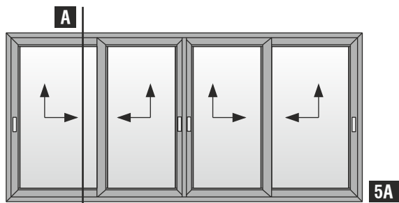
Τετράφυλλο φιλιτό επάλληλο ανασυρόμενο Four sash meeting stile parallel lift & slide
