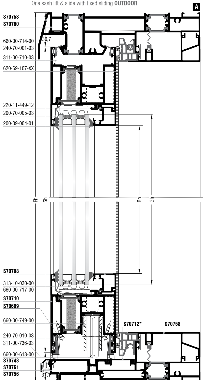
Μονόφυλλο ανασυρόμενο με σταθερά συρομένο ΕΞΩ One sash lift & slide with fixed sliding OUTDOOR
