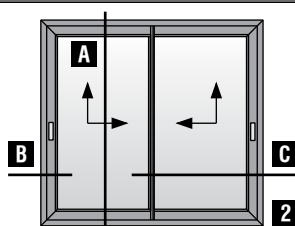
Δίφυλλο επάλληλο ανασυρόμενο παράθυρο (κοπή 90°) Two sash parallel lift & slide window (90° cutting)
