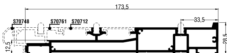
Προφίλ 1:2 | Profile 1:2
