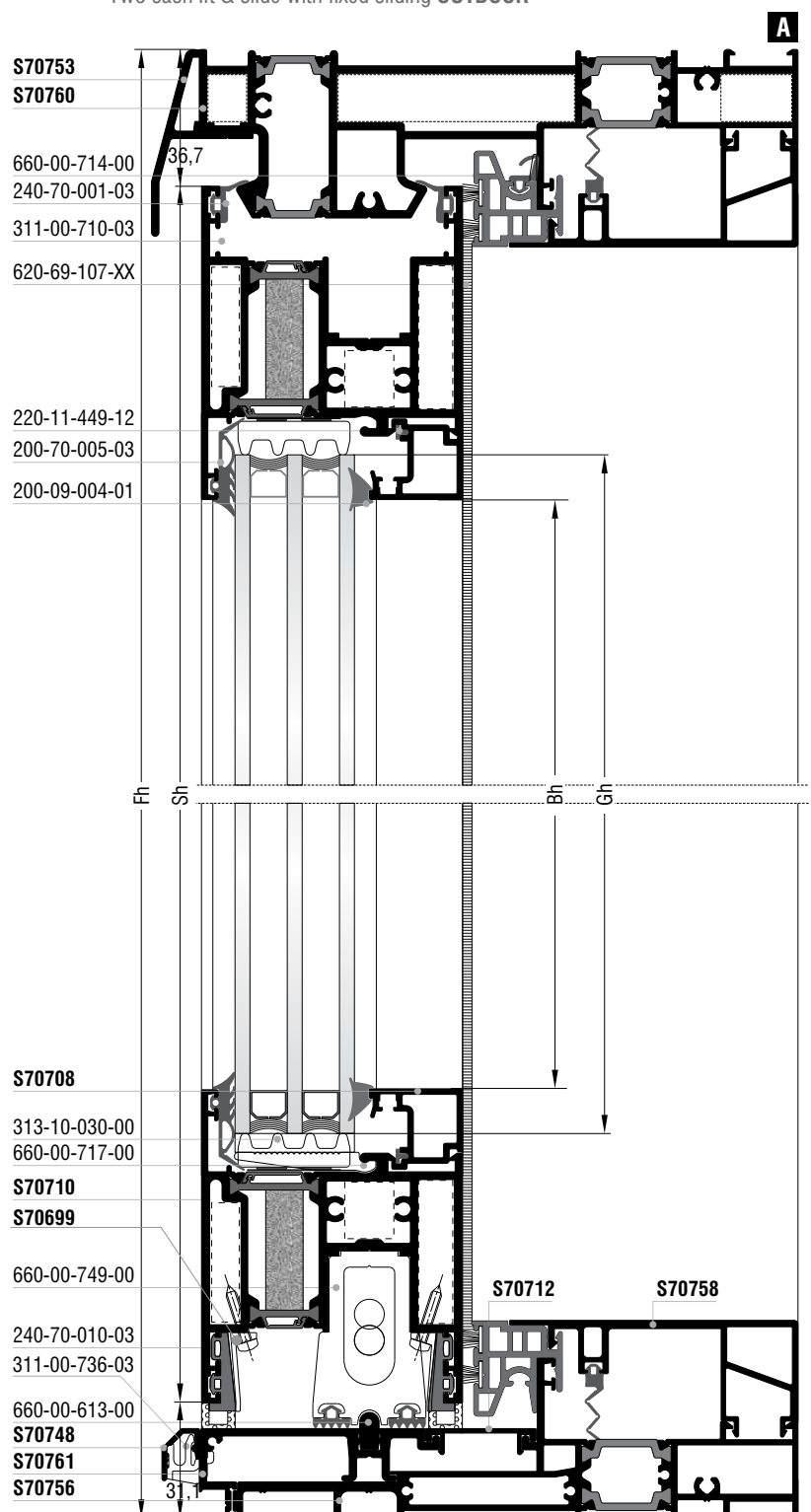
Δίφυλλο ανασυρόμενο με σταθερό συρόμενο ΕΞΩ Two sash lift & slide with fixed sliding OUTDOOR
