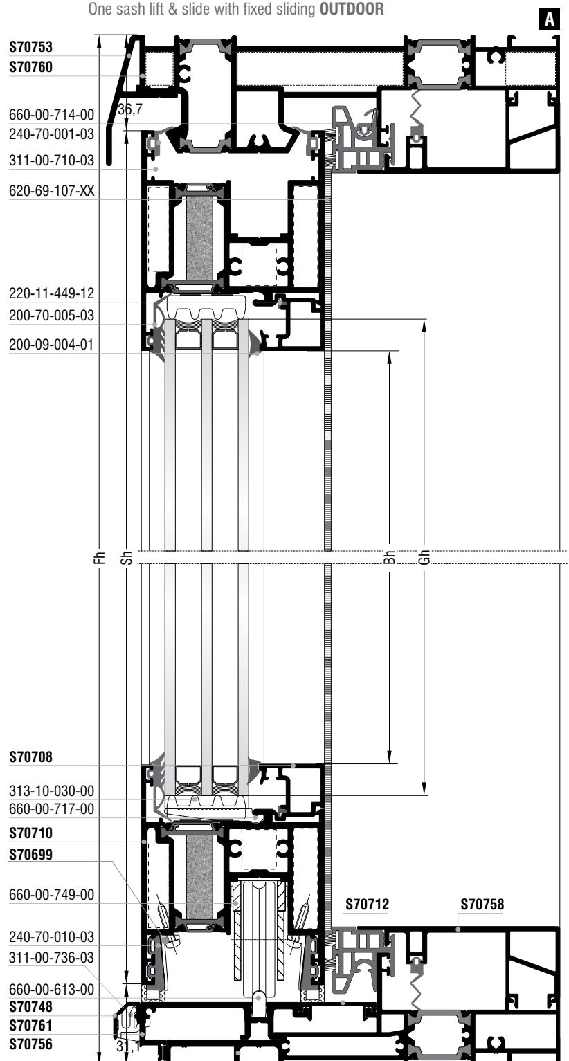
Μονόφυλλο ανασυρόμενο με σταθερά συρόμενο ΕΞΩ One sash lift & slide with fixed sliding OUTDOOR
