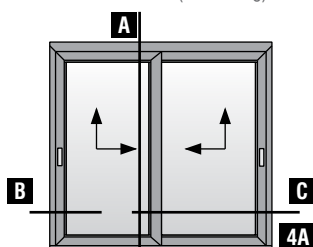
Δίφυλλο επάλληλο ανασυρόμενο ΔΕΞΙ με χρήση χαμηλού οδηγού S70786 Two sash parallel lift & slide RIGHT with S70786 short frame guide use
