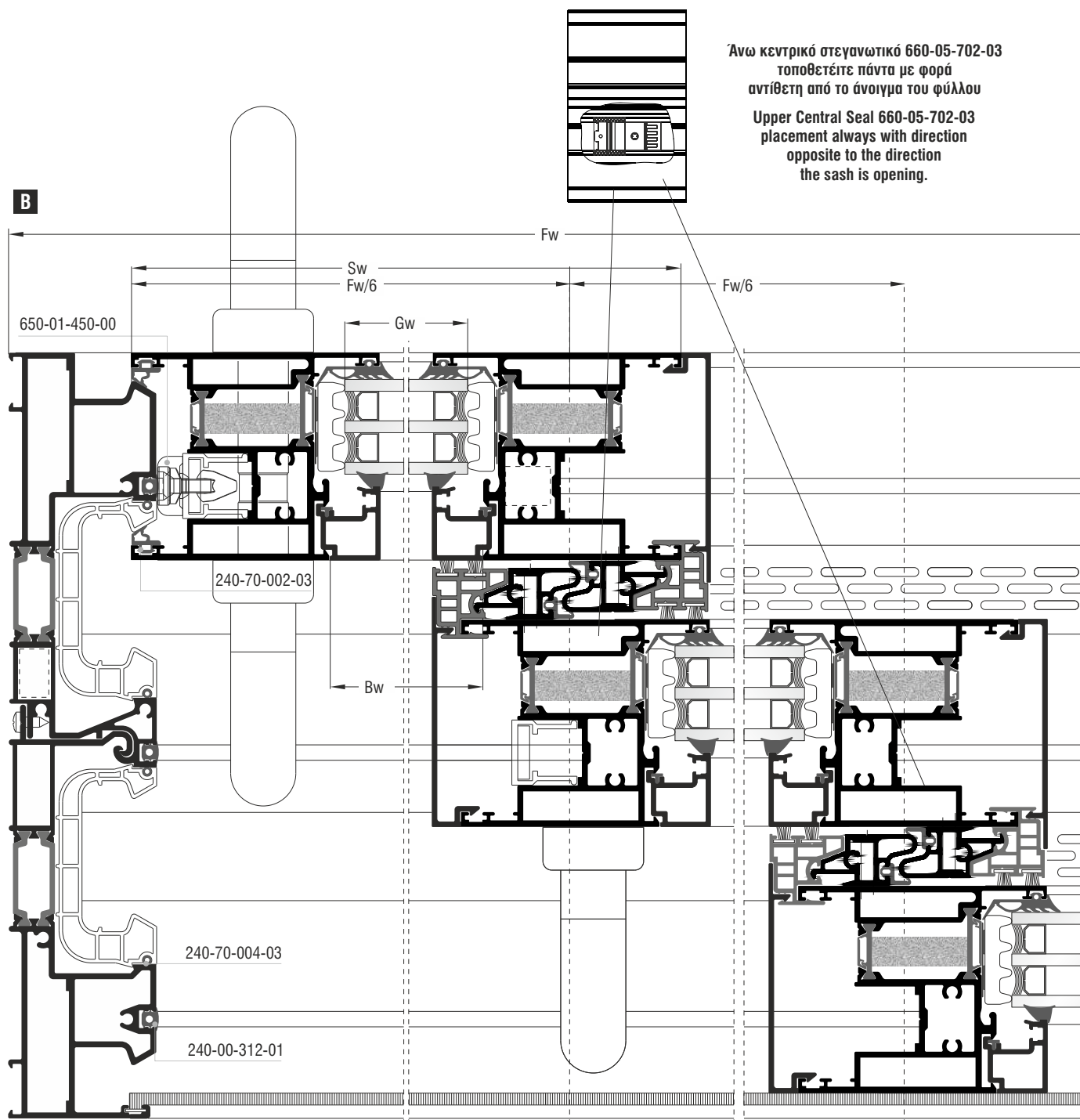
Εξάφυλλο επάλληλο φιλητό ανασυρόμενο με χρήση τριπλού οδηγού & χαμηλού οδηγού S70790 TPY Six sash parallel meeting stile lift & slide with tripleframe guide & S70790 TPY short frame guide use
