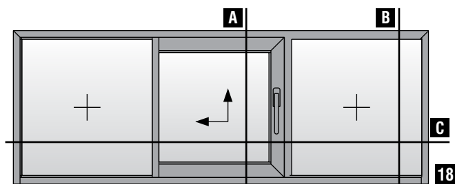
Μονόφυλλο ανασυρόμενο με σταθερά συρόμενο ΕΞΩ One sash lift & slide with fixed sliding OUTDOOR
