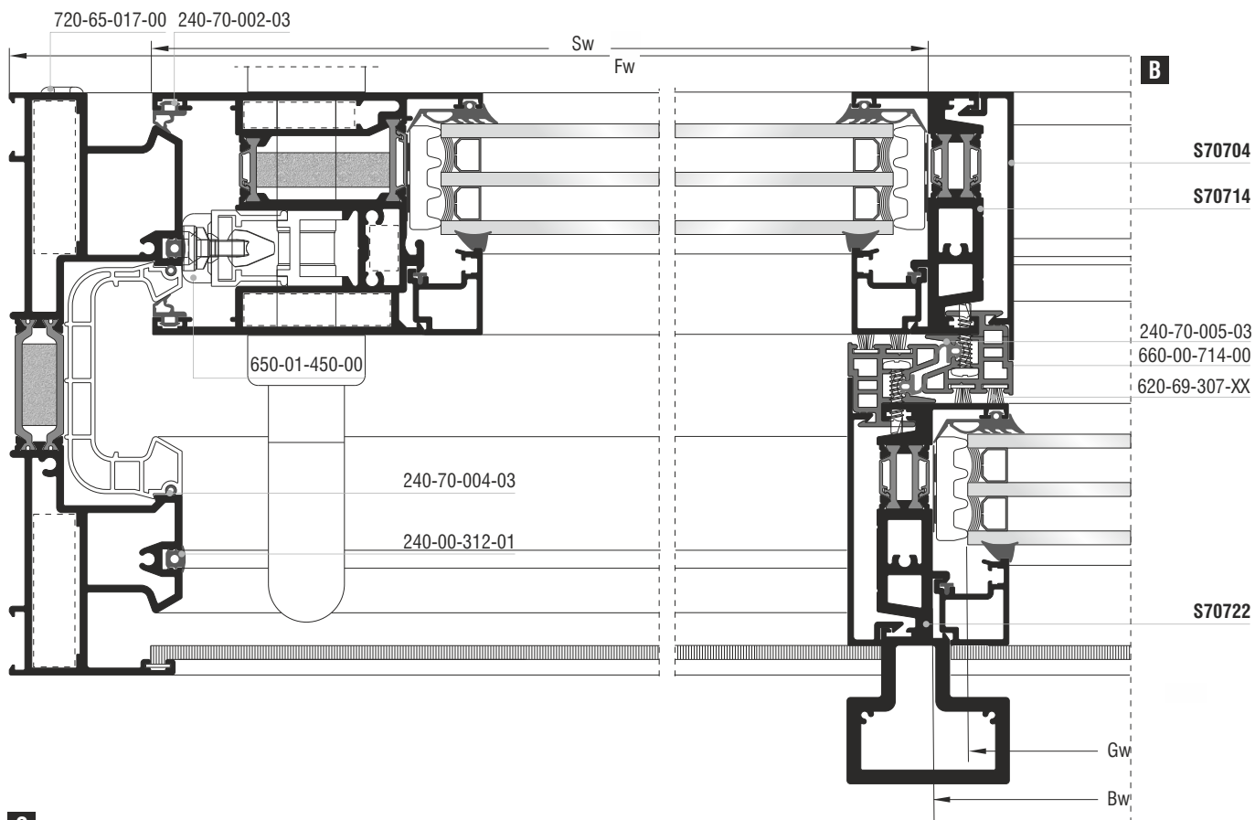
Τετράφυλλο φιλιτό επάλληλο ανασυρόμενο (κοπή 90°) Four sash meeting stile parallel lift & slide (90° cutting)
