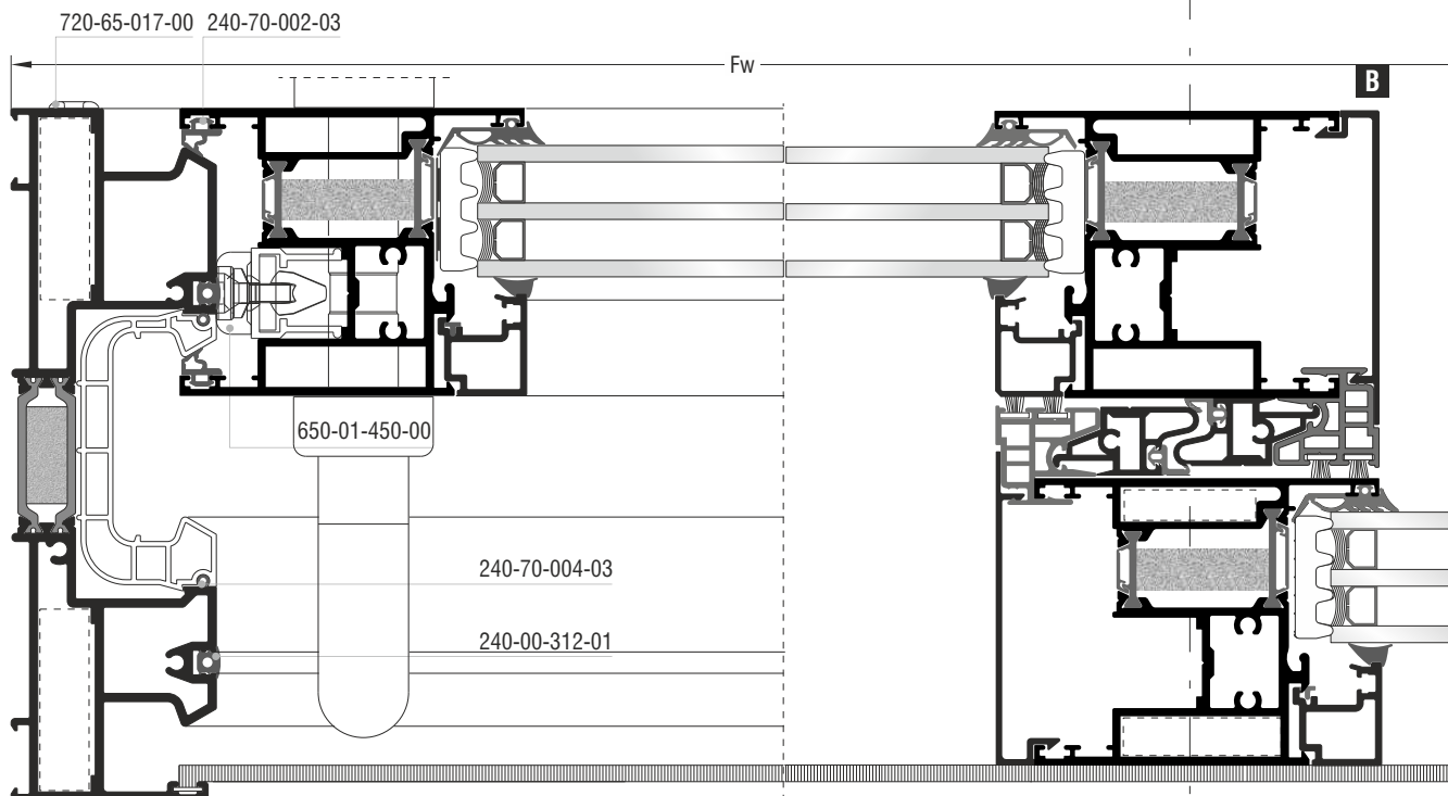
Τετράφυλλο φιλιτό επάλληλο ανασυρόμενο με χρήση χαμηλού οδηγού S70786 | Four sash parallel meeting stile lift & slide with S70786 short frame guide use
