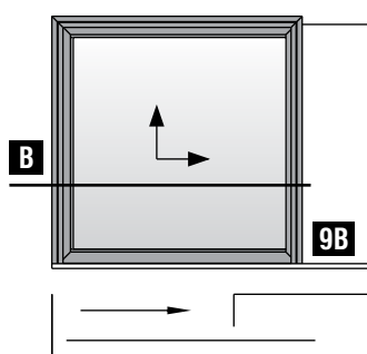
Μονόφυλλο χωνευτό δεξιά ανασυρόμενο παράθυρο One sash right pocket lift & slide window
