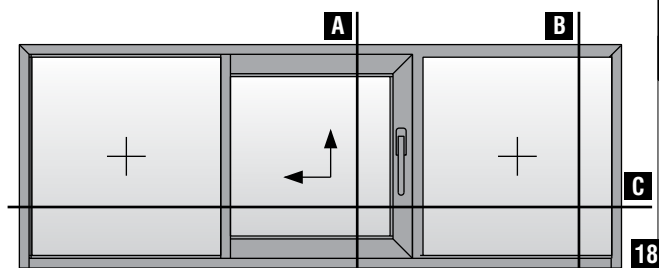
Μονόφυλλο ανασπώμενο με σταθερά συρόμενο ΕΞΩ One sash lift & slide with fixed sliding OUTDOOR
