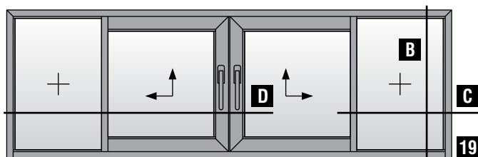
Δίφυλλο φιλητό αριστερά ανασυρόμενο με σταθερά συρόμενο ΕΞΩ Two sash meeting stile left lift & slide with fixed sliding OUTDOOR
