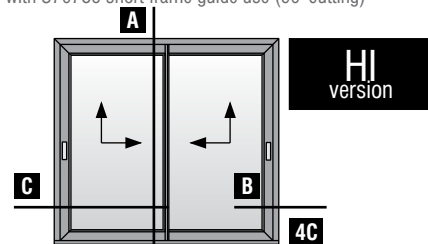
Δίφυλλο επάλληλο ανασυρόμενο ΔΕΞΙΟ με χρήση χαμηλού οδηγού S70786 και φύλλο S70776 Two sash parallel lift & slide RIGHT with S70786 short frame guide and S70776 sash use
