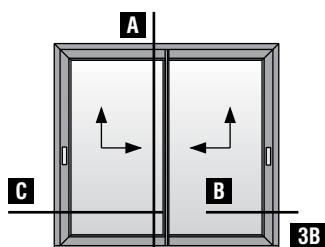
Δίφυλλο επάλληλο ανασυρόμενο ΑΡΙΣΤΕΡΟ με χρήση χαμηλού οδηγού S70786 (κοπή 90°) Two sash parallel lift & slide LEFT with S70786 short frame guide use (90° cutting)
