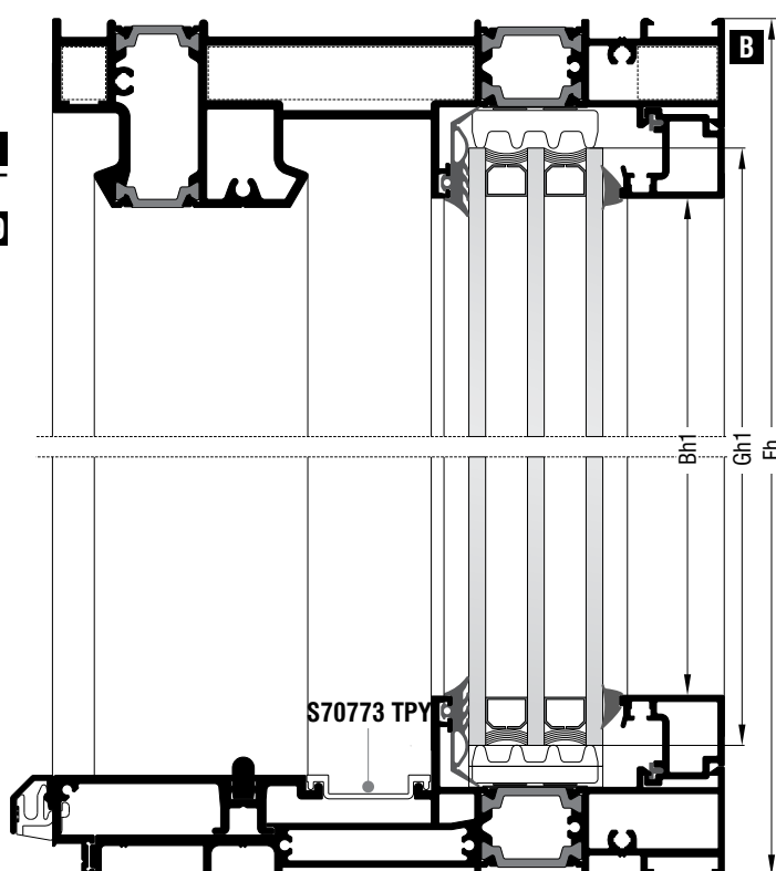
Δίφυλλο φιλητό αριστερά ανασυρόμενο με σταθερά συρόμενο ΕΞΩ Two sash meeting stile left lift & slide with fixed sliding OUTDOOR
