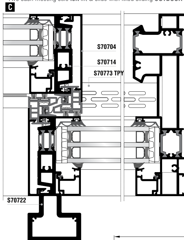
Δίφυλλο φιλητό αριστερά ανασυρόμενο με σταθερά συρόμενο ΕΞΩ Two sash meeting stile left lift & slide with fixed sliding OUTDOOR
