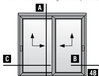
Δίφυλλο επάλληλο ανασυρόμενο ΑΡΙΣΤΕΡΟ με χρήση χαμηλού οδηγού S70786 Two sash parallel lift & slide LEFT with S70786 short frame guide use
