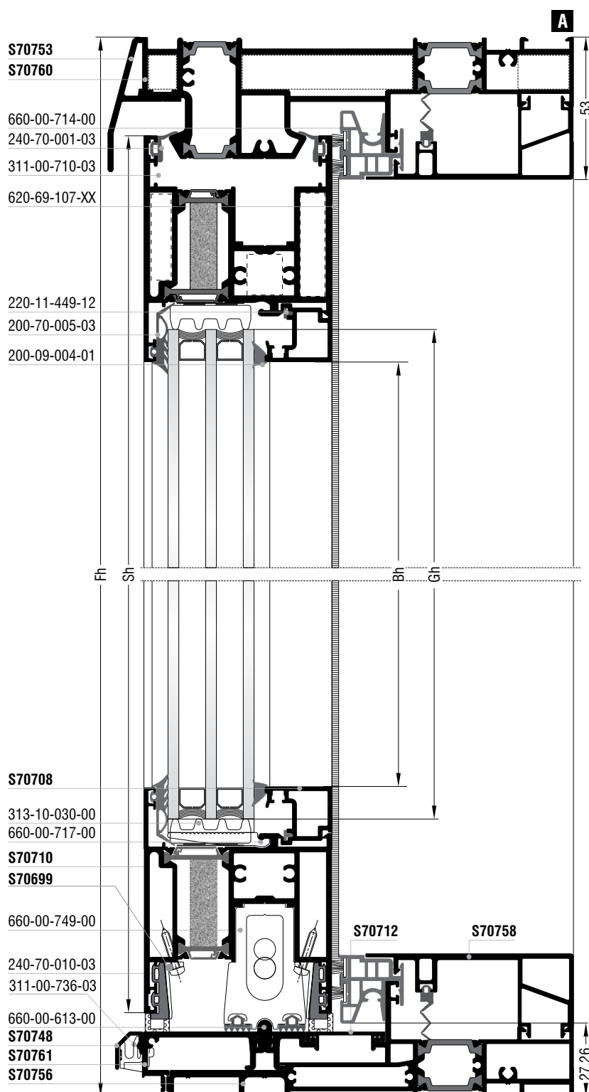
Δίφυλλο φιλητό αριστερά ανασυσρόμενο με σταθερά συρομένο ΕΞΩ Two sash meeting stile left lift & slide with fixed sliding OUTDOOR
