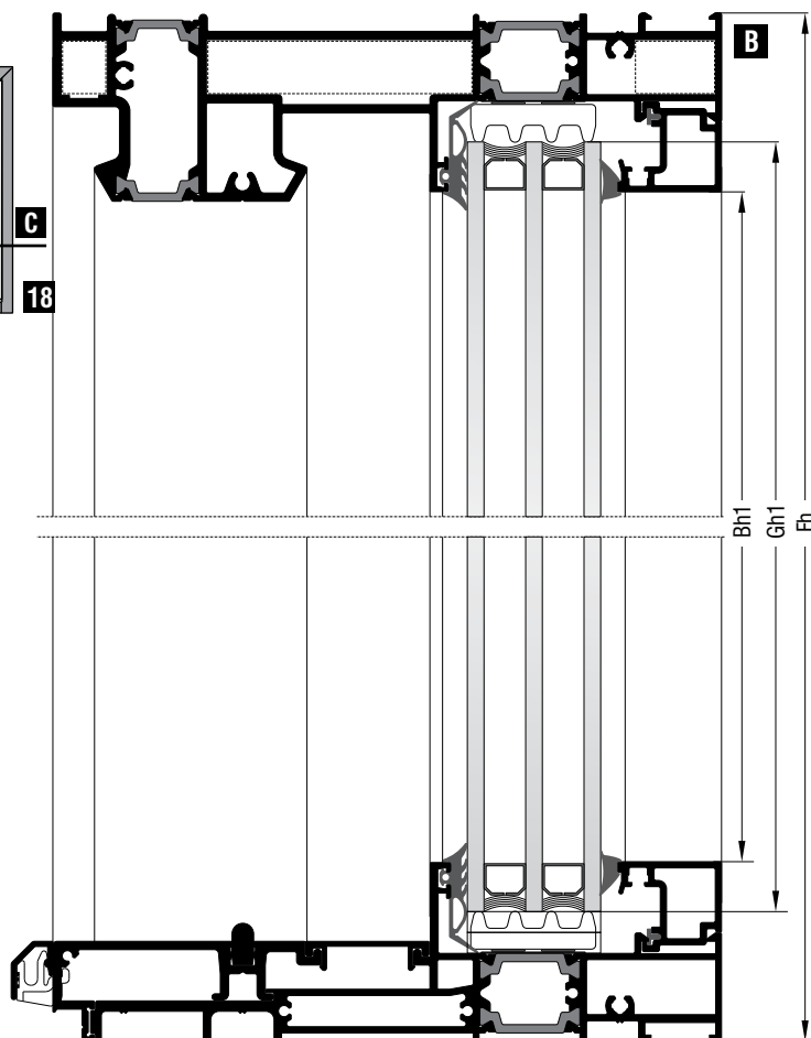
Μονόφυλλο ανασπώμενο με σταθερά συρόμενο ΕΞΩ One sash lift & slide with fixed sliding OUTDOOR
