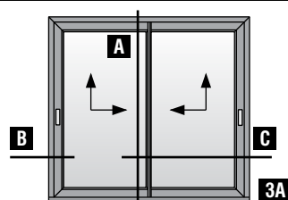
Δίφυλλο επάλληλο ανασυρόμενο ΔΕΞΙ με χρήση χαμηλού οδηγού S70786 (κοπή 90°) Two sash parallel lift & slide RIGHT with S70786 short frame guide use (90° cutting)
