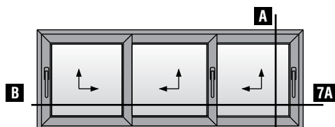
Τρίφυλλο επάλληλο ανασυρόμενο ΔΕΞΙ με χρήση χαμηλού οδηγού Three sash parallel lift & slide RIGHT with short frame guide use
