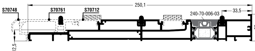
Προφίλ 1:2 | Profile 1:2
