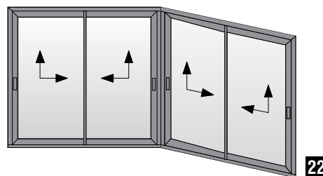
Τετράφυλλο επάλληλο (90° ΓΩΝΙΑ ΜΕΣΑ) γωνιακής συνεργασίας κοπή 90° με χαμηλό οδηγό και χαμηλό φύλλο Four sash parallel slide (90° INTERIOR CORNER ) (90° cutting), with short frame guide use and short sash
