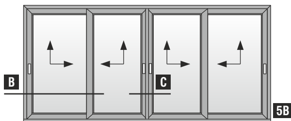
Τετράφυλλο φιλιτό επάλληλο ανασυρόμενο με χρήση χαμηλού οδηγού S70786 | Four sash parallel meeting stile lift & slide with S70786 short frame guide use
