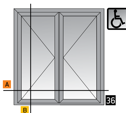
Double side-hung door inward opening without threshold Δίφυλλη πόρτα ανοιγόμενη μέσα με λάστιχο χωρίς κατωκάσι
