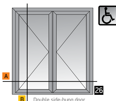
Double side-hung door inward opening without threshold Δίφυλλη πόρτα ανοιγομένη μέσα με λάστιχο χωρίς κατωκάσι
