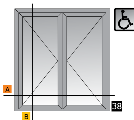
Double side-hung door inward opening with windbreak Δίφυλλη πόρτα ανοιγόμενη μέσα με ανεμοφράχτη
