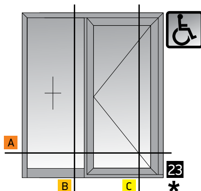
Single leaf entrance door opening inward with glass pane, one fixed side leaf Μονόφυλλη πόρτα εισόδου ανοιγομένη μέσα με υαλοπρίνα, ένα σταθερό
