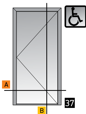
Single leaf door inward opening with windbreak Μονόφυλλη πόρτα ανοιγόμενη μέσα με ανεμοφράχτη
