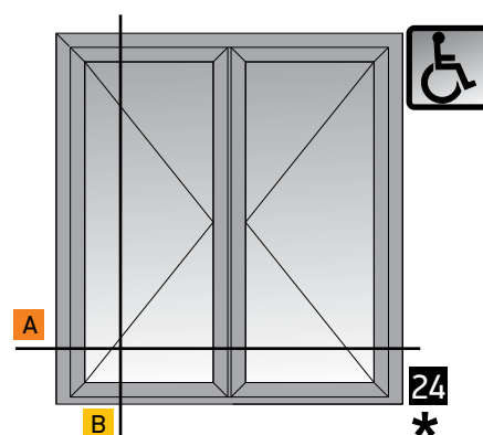
Double leaf entrance door opening inward with glass pane Δίφυλλη πόρτα εισόδου ανοιγομένη μέσα με υαλοπρίνα
