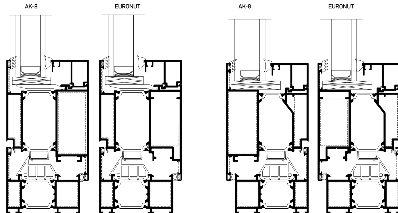
Hinges - Μεντεσέδες
