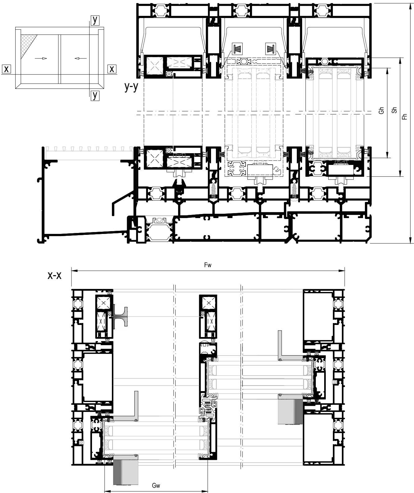
10 2Sash-3Track sliding window with flyscreen Δίφυλλο επάλληλο συρόμενο με σήτα
