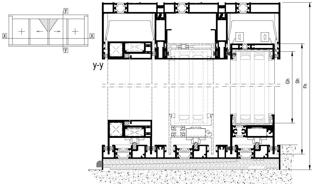
20 4Sashes with 2Fixed on 3-flat-track sliding window with flyscreen and meeting stile Τετράφυλλο φιλητό συρόμενο με συνεπίπεδο οδηγό, σήτα και σταθερά
