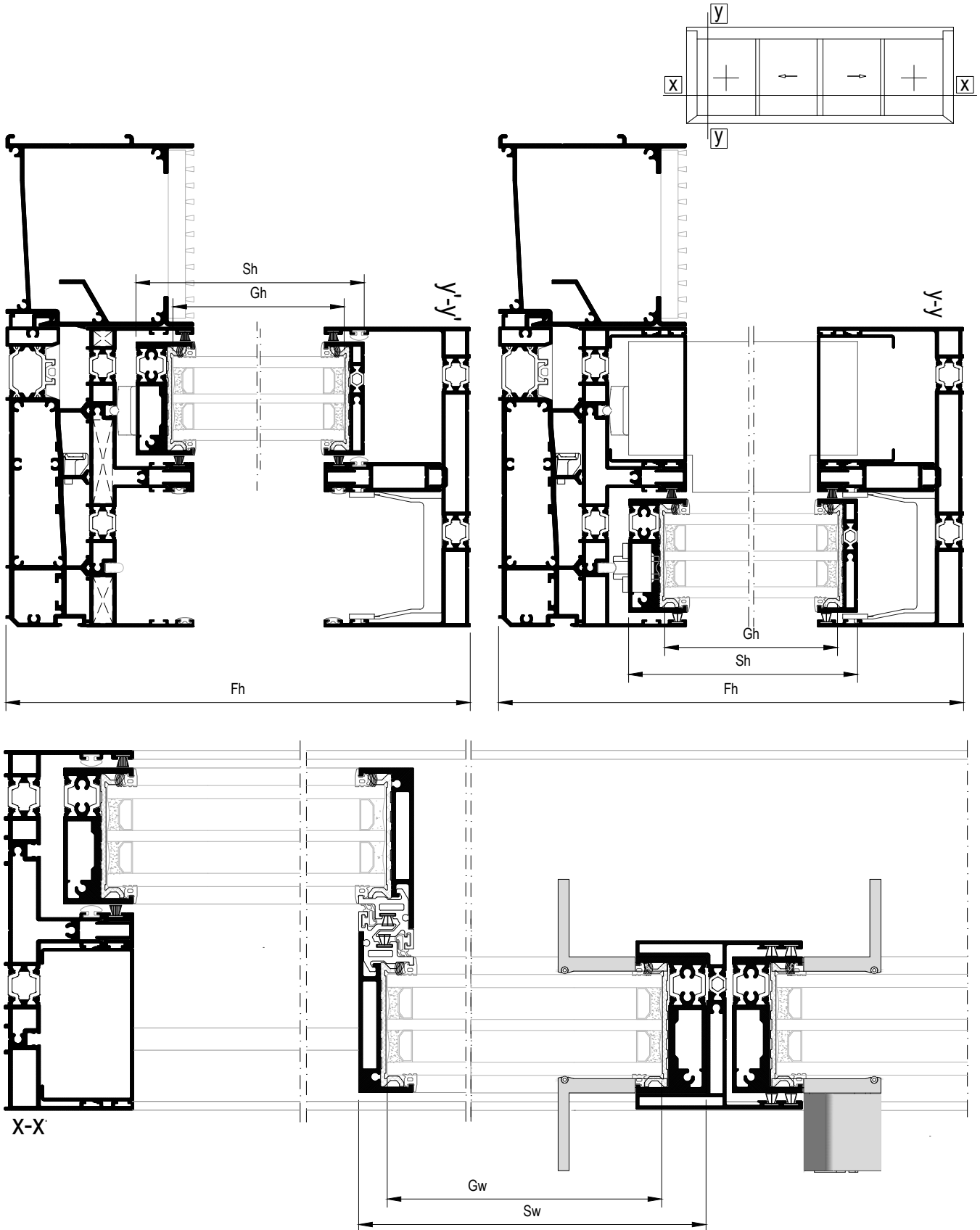
6 Four-sash sliding window with meeting stile and fixed Τετράφυλλο φιλητό συρόμενο με σταθερά
