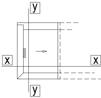
21 Single-sash pocket window Μονόφυλλο χωνευτό
