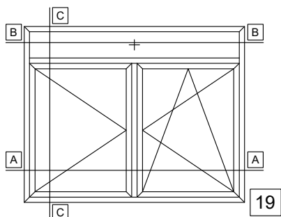
DOUBLE SIDE-HUNG CASEMENT TILT AND TURN WITH FIXED LIGHT ΜΟΝΟΦΥΛΛΟ ΑΝΟΙΓΟΜΕΝΟ-ΑΝΑΚΛΙΝΟΜΕΝΟ ΜΕ ΣΤΑΘΕΡΟ ΕΠΙΛΟΓ
