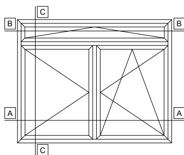
DOUBLE SIDE-HUNG CASEMENT TILT AND TURN WITH TILT LIGHT ΔΙΦΥΛΛΟ ΑΝΟΙΓΟΜΕΝΟ-ΑΝΑΚΛΙΝΟΜΕΝΟ ΜΕ ΦΕΓΓΙΤΗ
