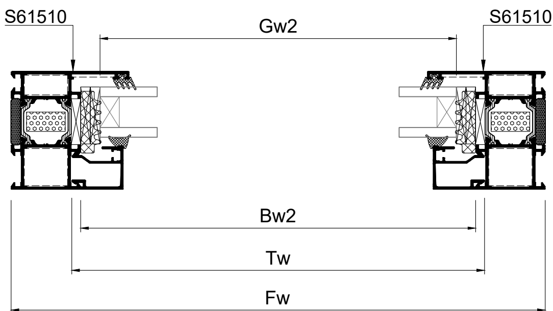
SINGLE SIDE-HUNG CASEMENT TILT AND TURN WITH FIXED LIGHT ΜΟΝΟΦΥΛΛΟ ΑΝΟΙΓΟΜΕΝΟ-ΑΝΑΚΛΙΝΟΜΕΝΟ ΜΕ ΣΤΑΘΕΡΟ ΕΓΓΛΩ
