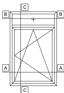
SINGLE SIDE-HUNG CASEMENT TILT AND TURN WITH FIXED LIGHT ΜΟΝΟΦΥΛΛΟ ΑΝΟΙΓΟΜΕΝΟ-ΑΝΑΚΛΙΝΟΜΕΝΟ ΜΕ ΣΤΑΘΕΡΟ ΕΓΓΛΩ
