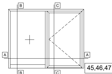
SINGLE SASH DOOR OUTWARD OPENING WITH FIXED SIDE PANEL ΜΟΝΟΦΥΛΛΗ ΠΟΡΤΑ ΑΝΟΙΓΟΜΕΝΗ ΕΞΩ ΜΕ ΕΝΑ ΣΤΑΘΕΡΟ
