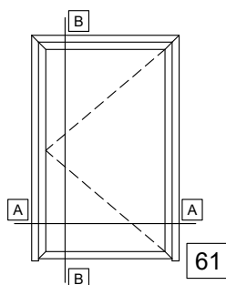
SINGLE SASH DOOR OUTWARD OPENING WITH WINDBREAK ΜΟΝΟΦΥΛΛΗ ΠΟΡΤΑ ΑΝΟΙΓΟΜΕΝΗ ΕΞΩ ΜΕ ΑΝΕΜΟΦΡΑΚΤΗ
