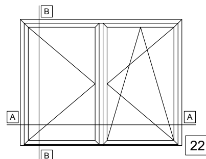
DOUBLE SIDE-HUNG CASEMENT TILT AND TURN WITH LOW THRESHOLD AND FOUR SASH SHUTTER WITHOUT THRESHOLD ΔΙΦΥΛΛΟ ΑΝΟΙΓΟΜΕΝΟ-ΑΝΑΚΛΙΝΟΜΕΝΟ ΜΕ ΧΑΜΗΛΟ ΚΑΤΩΚΑΣΙ ΚΑΙ ΤΕΤΡΑΦΥΛΛΟ ΠΑΝΤΖΟΥΡΙ ΧΩΡΙΣ ΚΑΤΩΚΑΣΙ
