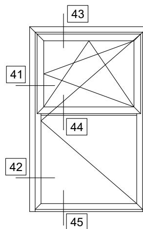
SINGLE SASH DOOR OPENING INWARD WITH INTEGRATED WINDOW ΜΟΝΟΦΥΛΛΗ ΠΟΡΤΑ ΑΝΟΙΓΟΜΕΝΗ ΜΕΣΑ ΜΕ ΕΝΣΩΜΑΤΩΜΕΝΟ ΠΑΡΑΘΥΡΟ
