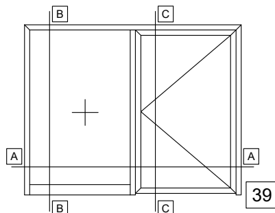
SINGLE SASH DOOR INWARD OPENING WITH FIXED SIDE PANEL WITH WINDBREAK ΜΟΝΟΦΥΛΛΗ ΠΟΡΤΑ ΑΝΟΙΓΟΜΕΝΗ ΜΕΣΑ ΜΕ ΕΝΑ ΣΤΑΘΕΡΟ ΜΕ ΑΝΕΜΟΦΡΑΚΤΗ
