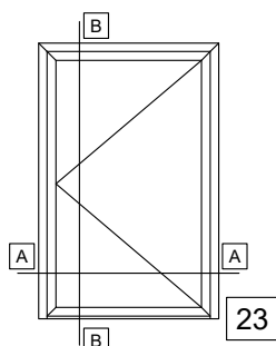
SINGLE SASH DOOR INWARD OPENING ΜΟΝΟΦΥΛΛΗ ΠΟΡΤΑ ΑΝΟΙΓΟΜΕΝΗ ΜΕΣΑ
