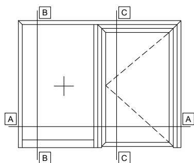
SINGLE SASH DOOR OUTWARD OPENING WITH FIXED SIDE PANEL WITHOUT THRESHOLD ΜΟΝΟΦΥΛΛΗ ΠΟΡΤΑ ΑΝΟΙΓΟΜΕΝΗ ΕΞΩ ΜΕ ΕΝΑ ΣΤΑΘΕΡΟ ΧΩΡΙΣ ΚΑΤΩΚΑΣΙ
