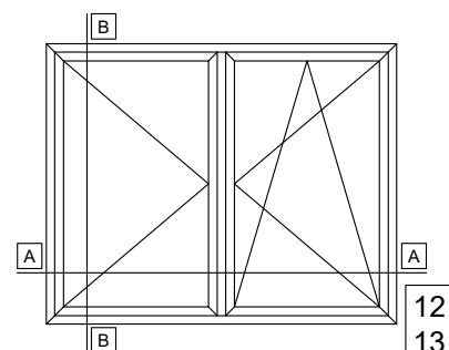
DOUBLE SIDE-HUNG CASEMENT TILT AND TURN WITH SHUTTER ΔΙΦΥΛΛΟ ΑΝΟΙΓΟΜΕΝΟ-ΑΝΑΚΛΙΝΟΜΕΝΟ ΜΕ ΠΑΝΤΖΟΥΡΙ
