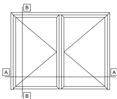
DOUBLE SASH DOOR INWARD OPENING WITH WINDBREAK ΔΙΦΥΛΛΗ ΠΟΡΤΑ ΑΝΟΙΓΟΜΕΝΗ ΜΕΣΑ ΜΕ ΑΝΕΜΟΦΡΑΚΤΗ
