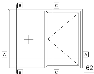
SINGLE SASH DOOR OUTWARD OPENING WITH FIXED SIDE PANEL WITH WINDBREAK ΜΟΝΟΦΥΛΛΗ ΠΟΡΤΑ ΑΝΟΙΓΟΜΕΝΗ ΕΞΩ ΜΕ ΕΝΑ ΣΤΑΘΕΡΟ ΜΕ ΑΝΕΜΟΦΡΑΚΤΗ
