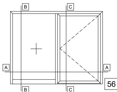
SINGLE SASH DOOR OUTWARD OPENING WITH FIXED SIDE PANEL ΜΟΝΟΦΥΛΛΗ ΠΟΡΤΑ ΑΝΟΙΓΟΜΕΝΗ ΕΞΩ ΜΕ ΕΝΑ ΣΤΑΘΕΡΟ
