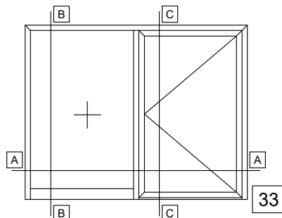
SINGLE SASH DOOR INWARD OPENING WITH FIXED SIDE PANEL ΜΟΝΟΦΥΛΛΗ ΠΟΡΤΑ ΑΝΟΙΓΟΜΕΝΗ ΜΕΣΑ ΜΕ ΕΝΑ ΣΤΑΘΕΡΟ
