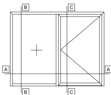
SINGLE SASH DOOR INWARD OPENING WITH FIXED SIDE PANEL ΜΟΝΟΦΥΛΛΗ ΠΟΡΤΑ ΑΝΟΙΓΟΜΕΝΗ ΜΕΣΑ ΜΕ ΕΝΑ ΣΤΑΘΕΡΟ
