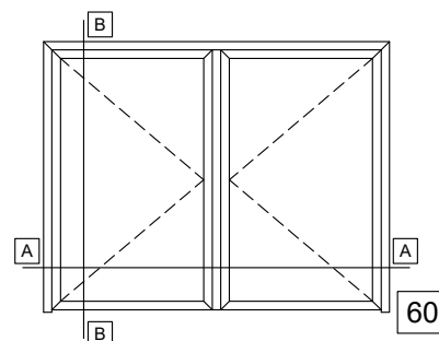
DOUBLE SASH DOOR OUTWARD OPENING WITHOUT THRESHOLD ΔΙΦΥΛΛΗ ΠΟΡΤΑ ΑΝΟΙΓΟΜΕΝΗ ΕΞΩ ΧΩΡΙΣ ΚΑΤΩΚΑΣΙ
