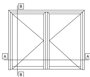
DOUBLE SASH DOOR INWARD OPENING WITH KICKPLATE ΔΙΦΥΛΛΗ ΠΟΡΤΑ ΑΝΟΙΓΟΜΕΝΗ ΜΕΣΑ ΜΕ ΤΑΜΠΛΑ
