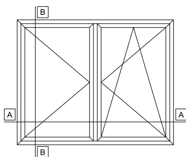
DOUBLE SIDE-HUNG CASEMENT TILT AND TURN WITH DOUBLE SASH SHUTTER ΔΙΦΥΛΛΟ ΑΝΟΙΓΟΜΕΝΟ-ΑΝΑΚΛΙΝΟΜΕΝΟ ΜΕ ΔΙΦΥΛΛΟ ΠΑΝΤΖΟΥΡΙ
