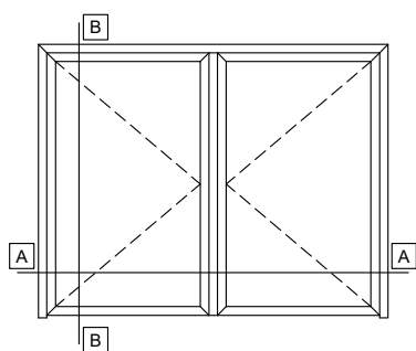
DOUBLE SASH DOOR OUTWARD OPENING WITH WINDBREAK ΔΙΦΥΛΛΗ ΠΟΡΤΑ ΑΝΟΙΓΟΜΕΝΗ ΕΞΩ ΜΕ ΑΝΕΜΟΦΡΑΚΤΗ
