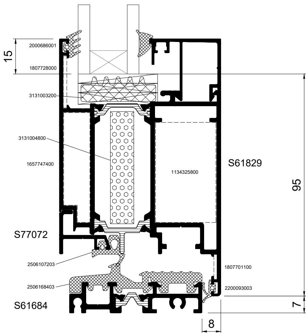
SINGLE SASH ENTRANCE DOOR OPENING INWARD ΜΟΝΟΦΥΛΛΗ ΠΟΡΤΑ ΕΙΣΟΔΟΥ ΑΝΟΙΓΟΜΕΝΗ ΜΕΣΑ
