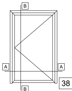
SINGLE SASH DOOR INWARD OPENING WITH WINDBREAK ΜΟΝΟΦΥΛΛΗ ΠΟΡΤΑ ΑΝΟΙΓΟΜΕΝΗ ΜΕΣΑ ΜΕ ΑΝΕΜΟΦΡΑΚΤΗ
