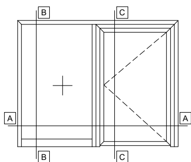
SINGLE SASH DOOR OUTWARD OPENING WITH FIXED SIDE PANEL WITH WINDBREAK ΜΟΝΟΦΥΛΛΗ ΠΟΡΤΑ ΑΝΟΙΓΟΜΕΝΗ ΕΞΩ ΜΕ ΕΝΑ ΣΤΑΘΕΡΟ ΜΕ ΑΝΕΜΟΦΡΑΚΤΗ
