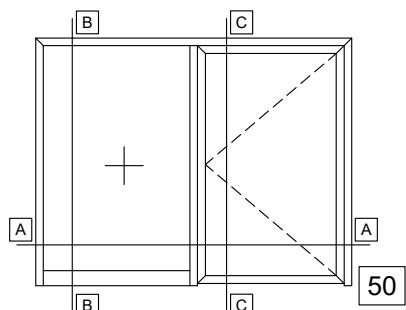
SINGLE SASH DOOR OUTWARD OPENING WITH FIXED SIDE PANEL WITHOUT THRESHOLD ΜΟΝΟΦΥΛΛΗ ΠΟΡΤΑ ΑΝΟΙΓΟΜΕΝΗ ΕΞΩ ΜΕ ΕΝΑ ΣΤΑΘΕΡΟ ΧΩΡΙΣ ΚΑΤΩΚΑΣΙ
