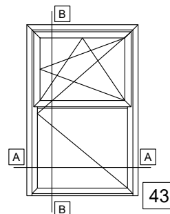
SINGLE SASH DOOR OPENING INWARD WITH INTEGRATED WINDOW ΜΟΝΟΦΥΛΛΗ ΠΟΡΤΑ ΑΝΟΙΓΟΜΕΝΗ ΜΕΣΑ ΜΕ ΕΝΣΩΜΑΤΩΜΕΝΟ ΠΑΡΑΘΥΡΟ
