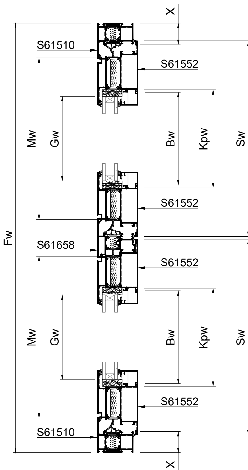
DOUBLE SASH DOOR INWARD OPENING WITH KICKPLATE ΔΙΦΥΛΛΗ ΠΟΡΤΑ ΑΝΟΙΓΟΜΕΝΗ ΜΕΣΑ ΜΕ ΤΑΜΠΛΑ
