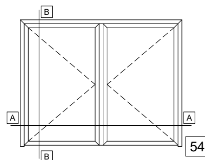
DOUBLE SASH DOOR OUTWARD OPENING WITH WINDBREAK ΔΙΦΥΛΛΗ ΠΟΡΤΑ ΑΝΟΙΓΟΜΕΝΗ ΕΞΩ ΜΕ ΑΝΕΜΟΦΡΑΚΤΗ
