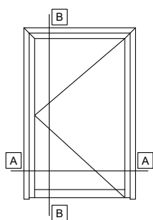
SINGLE SASH DOOR INWARD OPENING WITH KICKPLATE ΜΟΝΟΦΥΛΛΗ ΠΟΡΤΑ ΑΝΟΙΓΟΜΕΝΗ ΜΕΣΑ ΜΕ ΤΑΜΠΛΑ
