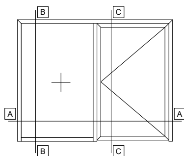
SINGLE SASH DOOR INWARD OPENING WITH FIXED SIDE PANEL WITH WINDBREAK ΜΟΝΟΦΥΛΛΗ ΠΟΡΤΑ ΑΝΟΙΓΟΜΕΝΗ ΜΕΣΑ ΜΕ ΕΝΑ ΣΤΑΘΕΡΟ ΜΕ ΑΝΕΜΟΦΡΑΚΤΗ
