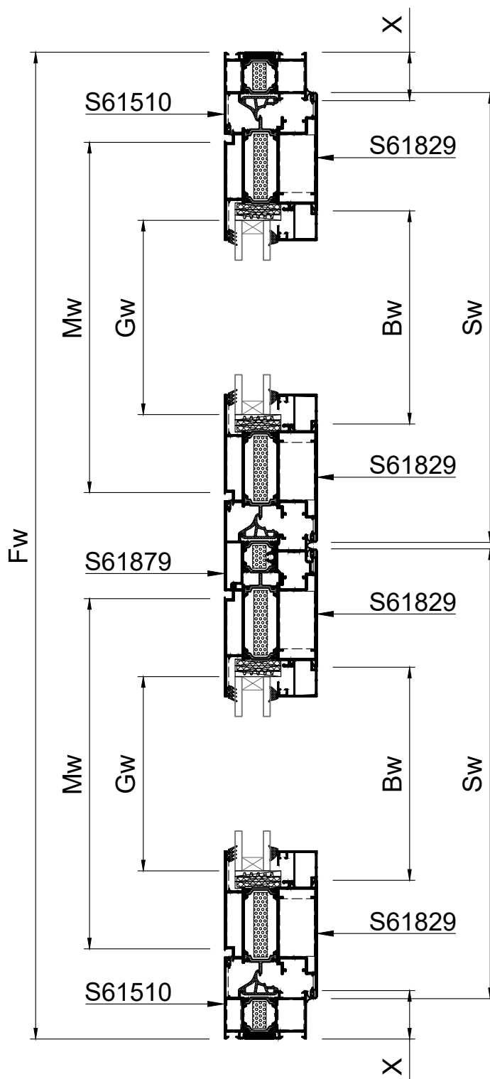
DOUBLE SASH DOOR INWARD OPENING WITH WINDBREAK ΔΙΦΥΛΛΗ ΠΟΡΤΑ ΑΝΟΙΓΟΜΕΝΗ ΜΕΣΑ ΜΕ ΑΝΕΜΟΦΡΑΚΤΗ
