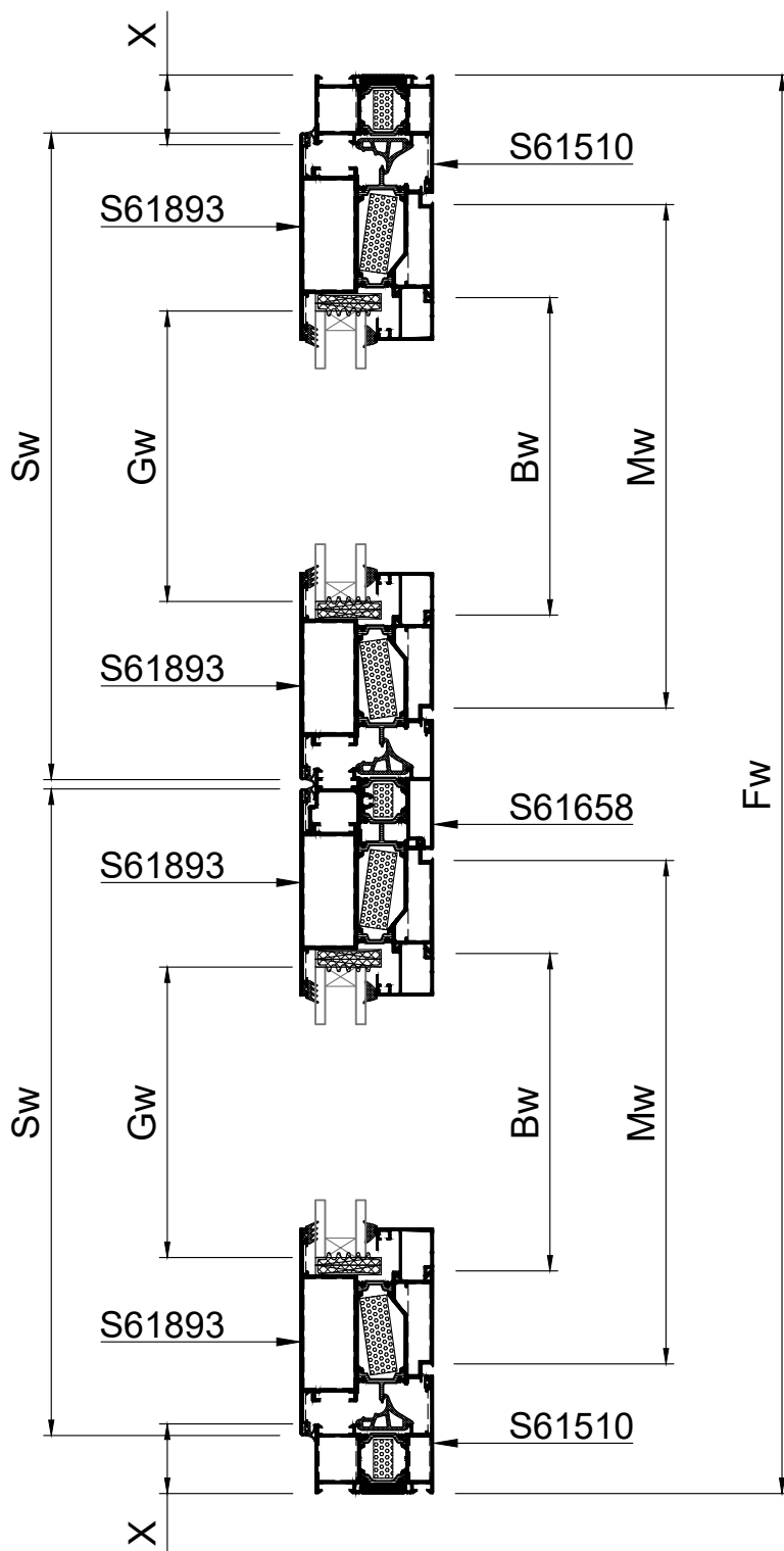
DOUBLE SASH DOOR OUTWARD OPENING WITH WINDBREAK ΔΙΦΥΛΛΗ ΠΟΡΤΑ ΑΝΟΙΓΟΜΕΝΗ ΕΞΩ ΜΕ ΑΝΕΜΟΦΡΑΚΤΗ
