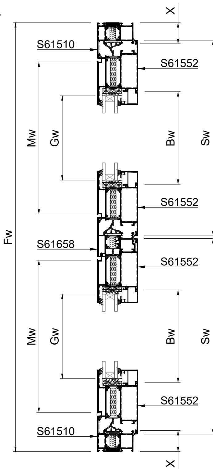
DOUBLE SASH DOOR INWARD OPENING WITHOUT THRESHOLD ΔΙΦΥΛΛΗ ΠΟΡΤΑ ΑΝΟΙΓΟΜΕΝΗ ΜΕΣΑ ΧΩΡΙΣ ΚΑΤΩΚΑΣΙ
