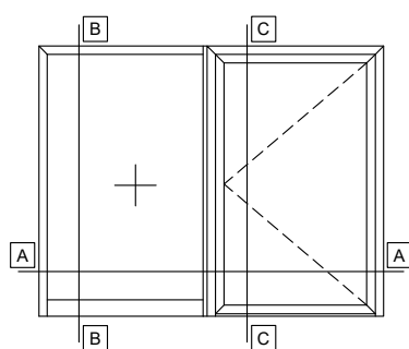
SINGLE SASH DOOR OUTWARD OPENING WITH FIXED SIDE PANEL ΜΟΝΟΦΥΛΛΗ ΠΟΡΤΑ ΑΝΟΙΓΟΜΕΝΗ ΕΞΩ ΜΕ ΕΝΑ ΣΤΑΘΕΡΟ
