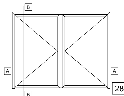
DOUBLE SASH DOOR INWARD OPENING WITHOUT THRESHOLD ΔΙΦΥΛΛΗ ΠΟΡΤΑ ΑΝΟΙΓΟΜΕΝΗ ΜΕΣΑ ΧΩΡΙΣ ΚΑΤΩΚΑΣΙ
