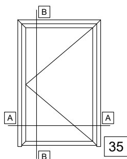
SINGLE SASH DOOR INWARD OPENING WITHOUT THRESHOLD ΜΟΝΟΦΥΛΛΗ ΠΟΡΤΑ ΑΝΟΙΓΟΜΕΝΗ ΜΕΣΑ ΧΩΡΙΣ ΚΑΤΩΚΑΣΙ
