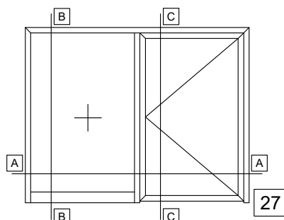
SINGLE SASH DOOR INWARD OPENING WITH FIXED SIDE PANEL WITHOUT THRESHOLD ΜΟΝΟΦΥΛΛΗ ΠΟΡΤΑ ΑΝΟΙΓΟΜΕΝΗ ΜΕΣΑ ΜΕ ΕΝΑ ΣΤΑΘΕΡΟ ΧΩΡΙΣ ΚΑΤΩΚΑΣΙ
