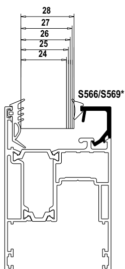
*S566 Powder coated colors- Ηλεκτροστατική βαφή S569 Ανοδίσωση-Anodising
