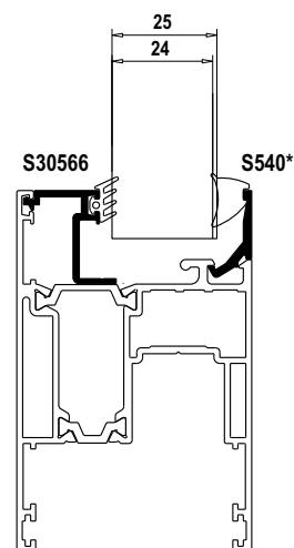
*S540 Powder coated colors- Ηλεκτροστατική βαφή
