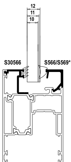
*S566 Powder coated colors- Ηλεκτροστατική βαφή S569 Ανοδίσωση-Anodising
