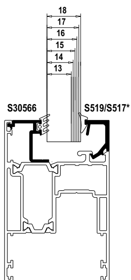
*S519 Powder coated colors- Ηλεκτροστατική βαφή S517 Ανοδίσωση-Anodising
