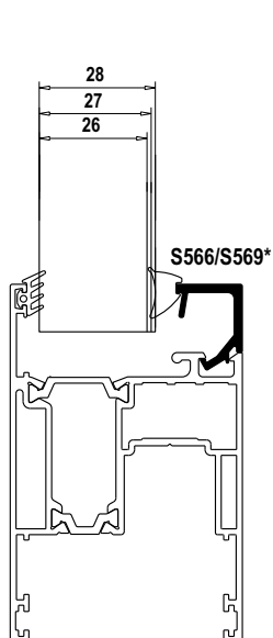
*S566 Powder coated colors- Ηλεκτροστατική βαφή S569 Ανοδίσωση-Anodising
