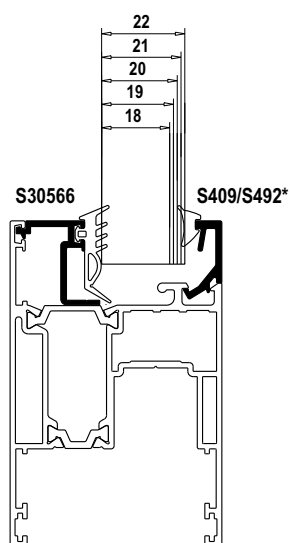
*S409 Powder coated colors- Ηλεκτροστατική βαφή S492 Ανοδίσωση-Anodising
