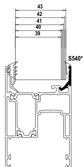
*S540 Powder coated colors- Ηλεκτροστατική βαφή
