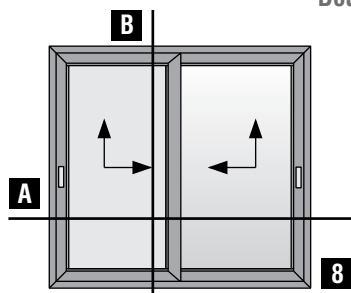
Δίφυλλο επάλληλο-ανασυρόμενο παράθυρο Με χρήση μόνο μεγάλου φύλλου S584 Double sash parallel lift & slide window Large sash use S584 only
