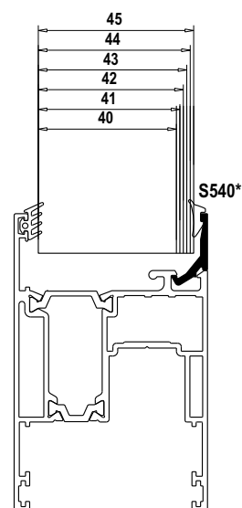
*S540 Powder coated colors- Ηλεκτροστατική βαφή
