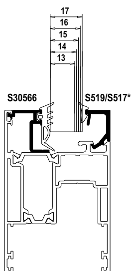
*S519 Powder coated colors- Ηλεκτροστατική βαφή S517 Ανοδίσωση-Anodising
