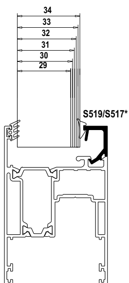
*S519 Powder coated colors- Ηλεκτροστατική βαφή S517 Ανοδίσωση-Anodising
