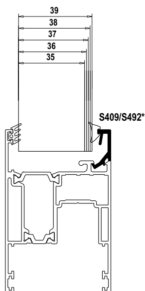
*S409 Powder coated colors- Ηλεκτροστατική βαφή S492 Ανοδίσωση-Anodising
