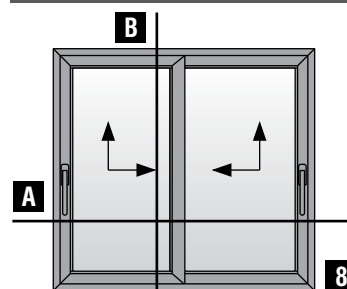
Δίφυλλο επάλληλο-ανασυρόμενο παράθυρο Με χρήση μόνο μεγάλου φύλλου S584 Double sash parallel lift & slide window Large sash use only S584
