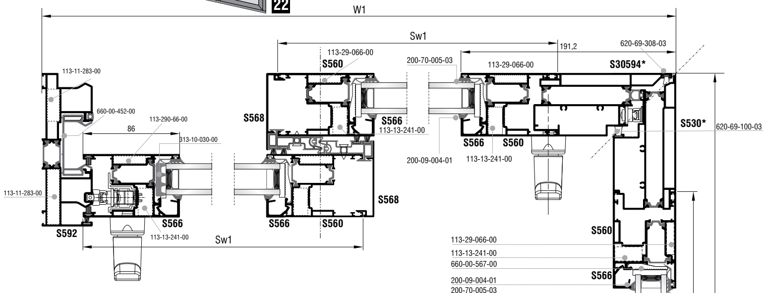
Τετράφυλλο επάλληλο (ΓΩΝΙΑ ΕΞΩ) γωνιακής συνεργασίας Corner assembly with four sash parallel slide (EXTERIOR CORNER)
