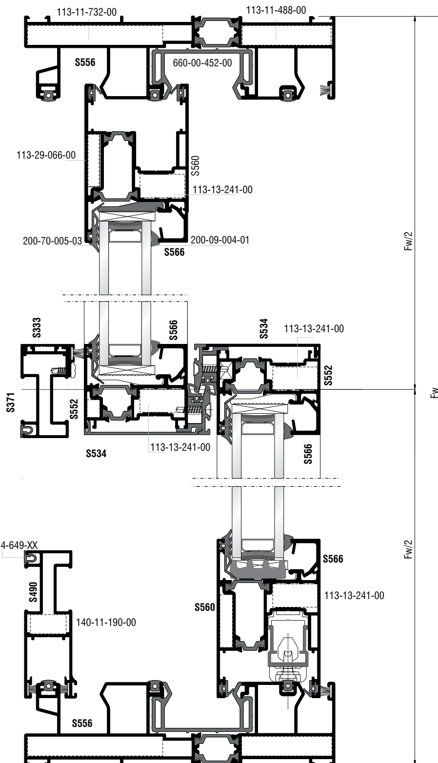
Δίφυλλο επάλληλο ανασυρόμενο παράθυρο με στενό γάντζο και σήτα Double sash parallel lift & slide window with narrow interlocking profile and fly-screen
