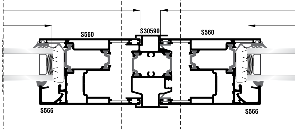
Δίφυλλο φιλητό ανασυρόμενο με σταθερά Double sash meeting stile lift & slide with fixed panes
