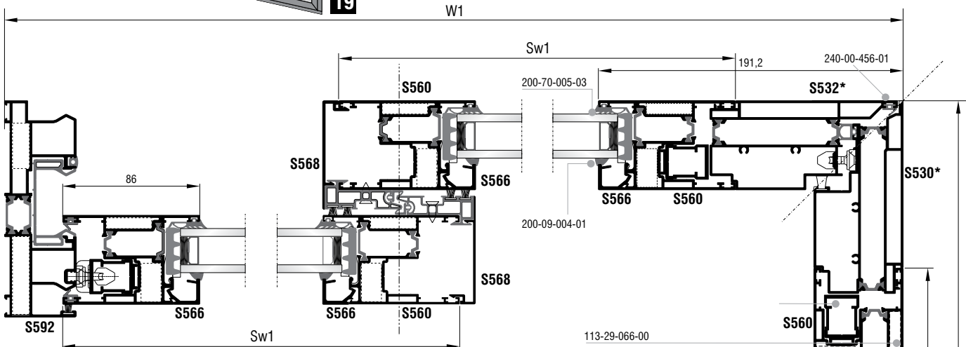
Τετράφυλλο επάλληλο (ΓΩΝΙΑ ΕΞΩ) γωνιακής συνεργασίας Corner assembly with four sash parallel slide (EXTERIOR CORNER)
