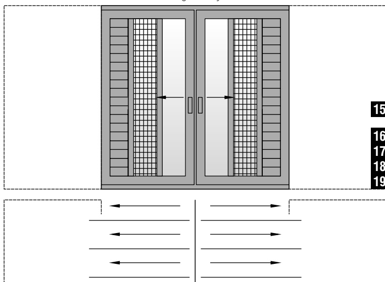
Δίφυλλο χωνευτό συρόμενο με σήτα & παντζούρι Two sash wall sliding with fly-screen & shutter
