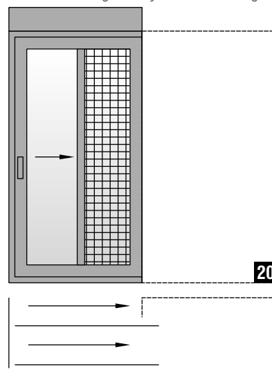
Μονόφυλλο χωνευτό συρόμενο με σήτα & ρολό One sash wall sliding with fly-screen & rolling shutter
