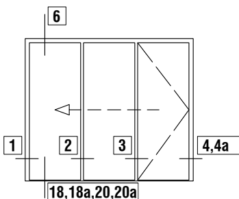
INWARD OPENING 3 PANELS ON ONE SIDE FOLDING DOOR ΕΞΩ ΑΝΟΙΓΟΜΕΝΗ 3 ΦΥΛΛΗ ΦΥΣΟΥΝΑ ΣΕ ΜΙΑ ΠΛΕΥΡΑ
