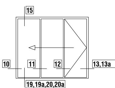
INWARD OPENING 3 PANELS ON ONE SIDE FOLDING DOOR LOW THRESHOLD ΕΞΩ ΑΝΟΙΓΟΜΕΝΗ 3 ΦΥΛΛΗ ΦΥΣΟΥΝΑ ΣΕ ΜΙΑ ΠΛΕΥΡΑ ΧΑΜΗΛΟ ΚΑΤΩΚΑΣΙ
