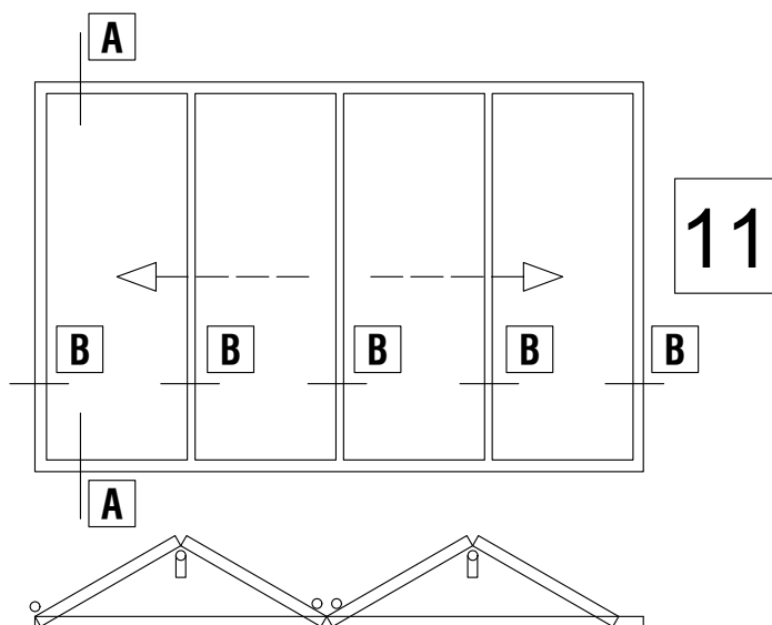
OUTWARD OPENING 2+2 4-PANELS ON ONE SIDE FOLDING DOOR ΕΞΩ ΑΝΟΙΓΟΜΕΝΗ 2+2 4-ΦΥΛΛΗ ΦΥΣΟΥΝΑ ΣΕ ΜΙΑ ΠΛΕΥΡΑ
