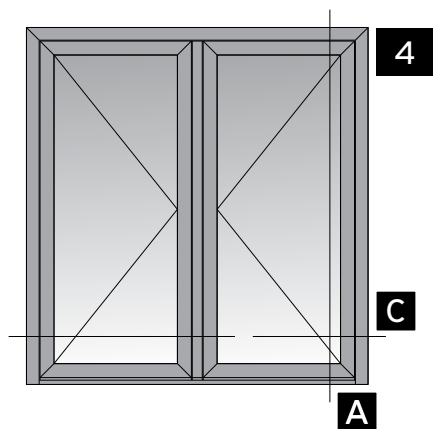
Double sash entrance door opening inward with glass panel with 15mm threshold Δίφυλλη πόρτα εισόδου ανοιγομένη μέσα με υαλοπίνακα και κατωκάσι 15mm
