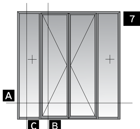
Double sash entrance door opening inward with glass panel, two fixed sash with transom Δίφυλλη πόρτα εισόδου ανοιγομένη μέσα με υαλοπίνακα, δύο σταθερά εκατέρωθεν και ταν
