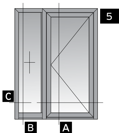
Single sash entrance door opening inward with glass panel, one fixed side sash and continuous threshold Μονόφυλλη πόρτα εισόδου ανοιγομένη μέσα με υαλοπίνακα, ένα σταθερό και ενιαίο κατωκάσι
