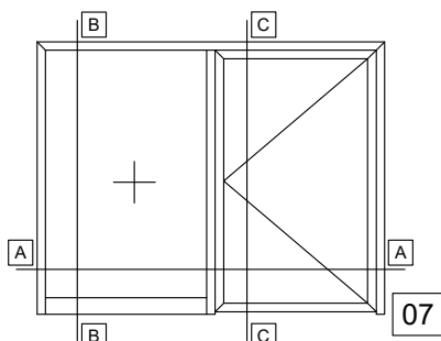
07 SINGLE LEAF DOOR INWARD OPENING WITH GLASS PANEL, WITHOUT THRESHOLD AND ONE FIXED SIDE PANEL WITH TRANSOM AND KICKPLATE ΜΟΝΟΦΥΛΛΗ ΠΟΡΤΑ ΑΝΟΙΓΟΜΕΝΗ ΜΕΣΑ ΜΕ ΥΑΛΟΠΙΝΑΚΑ, ΧΩΡΙΣ ΚΑΤΩΚΑΣΙ ΚΑΙ ΕΝΑ ΣΤΑΘΕΡΟ ΜΕ ΤΑΥ ΚΑΙ ΤΑΜΠΛΑ
