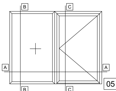
05 SINGLE LEAF DOOR INWARD OPENING WITH GLASS PANEL, WITH LOW THRESHOLD AND ONE FIXED SIDE PANEL ΜΟΝΟΦΥΛΛΗ ΠΟΡΤΑ ΑΝΟΙΓΟΜΕΝΗ ΜΕΣΑ ΜΕ ΥΑΛΟΠΙΝΑΚΑ, ΜΕ ΧΑΜΗΛΟ ΚΑΤΩΚΑΣΙ ΚΑΙ ΕΝΑ ΑΝΕΞΑΡΤΗΤΟ ΣΤΑΘΕΡΟ
