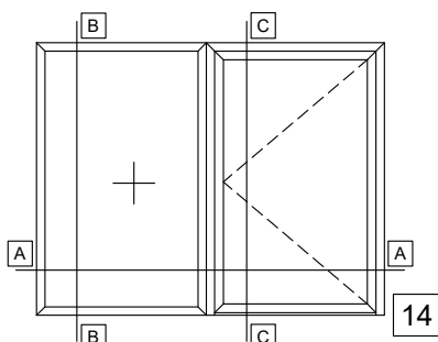
SINGLE LEAF DOOR INWARD OPENING WITH GLASS PANEL, WITH LOW THRESHOLD AND ONE FIXED SIDE PANEL WITH KICKPLATE ΜΟΝΟΦΥΛΛΗ ΠΟΡΤΑ ΑΝΟΙΓΟΜΕΝΗ ΜΕΣΑ ΜΕ ΥΑΛΟΠΙΝΑΚΑ, ΜΕ ΧΑΜΗΛΟ ΚΑΤΩΚΑΣΙ ΚΑΙ ΕΝΑ ΑΝΕΞΑΡΤΗΤΟ ΣΤΑΘΕΡΟ
