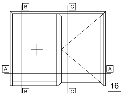
SINGLE LEAF DOOR INWARD OPENING WITH GLASS PANEL, WITHOUT THRESHOLD AND ONE FIXED SIDE PANEL WITH TRANSOM AND KICKPLATE ΜΟΝΟΦΥΛΛΗ ΠΟΡΤΑ ΑΝΟΙΓΟΜΕΝΗ ΜΕΣΑ ΜΕ ΥΑΛΟΠΙΝΑΚΑ, ΧΩΡΙΣ ΚΑΤΩΚΑΣΙ ΚΑΙ ΕΝΑ ΣΤΑΘΕΡΟ ΜΕ ΤΑΥ ΚΑΙ ΤΑΜΠΛΑ
