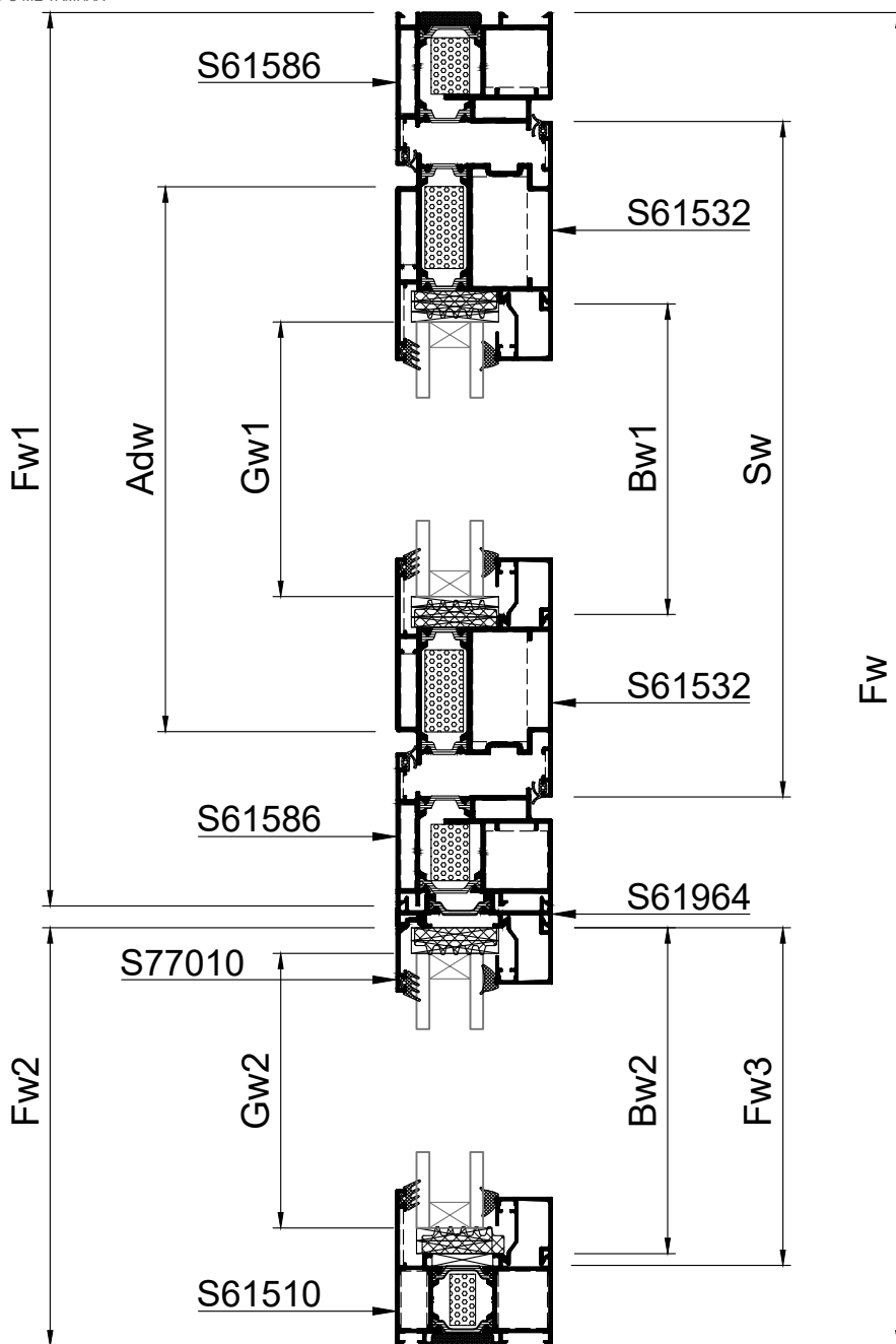
SINGLE LEAF DOOR INWARD OPENING WITH GLASS PANEL, WITHOUT THRESHOLD AND ONE FIXED SIDE PANEL WITH KICKPLATE ΜΟΝΟΦΥΛΛΗ ΠΟΡΤΑ ΑΝΟΙΓΟΜΕΝΗ ΜΕΣΑ ΜΕ ΥΑΛΟΠΙΝΑΚΑ, ΧΩΡΙΣ ΚΑΤΩΚΑΣΙ ΚΑΙ ΕΝΑ ΣΤΑΘΕΡΟ ΜΕ ΤΑΜΠΛΑ
