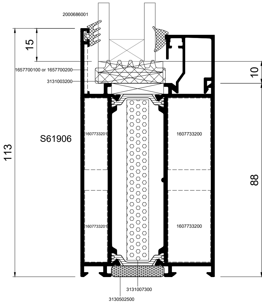
SINGLE LEAF ENTRANCE DOOR OPENING INWARD WITH FIXED SIDE ΜΟΝΟΦΥΛΛΗ ΠΟΡΤΑ ΕΙΣΟΔΟΥ ΑΝΟΙΓΟΜΕΝΗ ΜΕΣΑ ΜΕ ΣΤΑΘΕΡΟ
