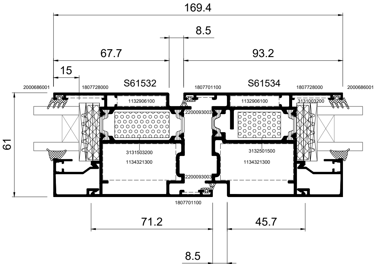
DOUBLE LEAF ENTRANCE DOOR OPENING OUTWARD ΔΙΦΥΛΛΗ ΠΟΡΤΑ ΕΙΣΟΔΟΥ ΑΝΟΙΓΟΜΕΝΗ ΕΞΩ
