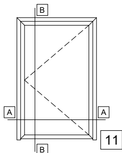
SINGLE LEAF DOOR INWARD OPENING WITH GLASS PANEL, WITHOUT THRESHOLD ΜΟΝΟΦΥΛΛΗ ΠΟΡΤΑ ΑΝΟΙΓΟΜΕΝΗ ΜΕΣΑ ΜΕ ΥΑΛΟΠΙΝΑΚΑ, ΧΩΡΙΣ ΚΑΤΩΚΑΣΙ
