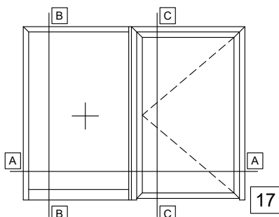
SINGLE LEAF DOOR INWARD OPENING WITH GLASS PANEL, WITHOUT THRESHOLD AND ONE FIXED SIDE PANEL WITH KICKPLATE ΜΟΝΟΦΥΛΛΗ ΠΟΡΤΑ ΑΝΟΙΓΟΜΕΝΗ ΜΕΣΑ ΜΕ ΥΑΛΟΠΙΝΑΚΑ, ΧΩΡΙΣ ΚΑΤΩΚΑΣΙ ΚΑΙ ΕΝΑ ΣΤΑΘΕΡΟ ΚΑΙ ΤΑΜΠΛΑ
