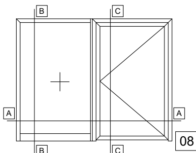
08 SINGLE LEAF DOOR INWARD OPENING WITH GLASS PANEL, WITHOUT THRESHOLD AND ONE FIXED SIDE PANEL WITH KICKPLATE ΜΟΝΟΦΥΛΛΗ ΠΟΡΤΑ ΑΝΟΙΓΟΜΕΝΗ ΜΕΣΑ ΜΕ ΥΑΛΟΠΙΝΑΚΑ, ΧΩΡΙΣ ΚΑΤΩΚΑΣΙ ΚΑΙ ΕΝΑ ΣΤΑΘΕΡΟ ΚΑΙ ΤΑΜΠΛΑ
