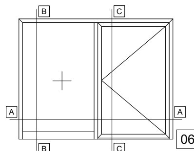
06 SINGLE LEAF DOOR INWARD OPENING WITH GLASS PANEL, WITH LOW THRESHOLD AND ONE FIXED SIDE PANEL WITH TRANSOM AND KICKPLATE ΜΟΝΟΦΥΛΛΗ ΠΟΡΤΑ ΑΝΟΙΓΟΜΕΝΗ ΜΕΣΑ ΜΕ ΥΑΛΟΠΙΝΑΚΑ, ΜΕ ΧΑΜΗΛΟ ΚΑΤΩΚΑΣΙ ΚΑΙ ΕΝΑ ΣΤΑΘΕΡΟ ΜΕ ΤΑΥ ΚΑΙ ΤΑΜΠΛΑ
