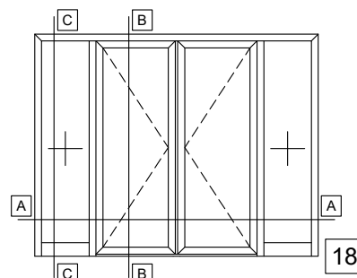
DOUBLE LEAF DOOR INWARD OPENING WITH GLASS PANEL, WITH TWO FIXED SIDE PANELS ΔΙΦΥΛΛΗ ΠΟΡΤΑ ΑΝΟΙΓΟΜΕΝΗ ΜΕΣΑ ΜΕ ΥΑΛΟΠΙΝΑΚΑ, ΜΕ ΔΥΟ ΣΤΑΘΕΡΑ ΕΚΑΤΕΡΩΘΕΝ
