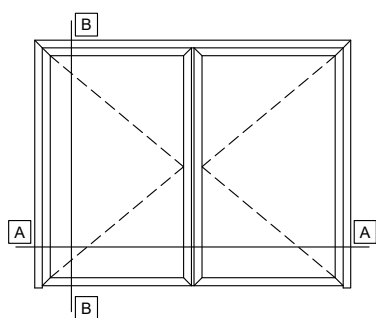
DOUBLE LEAF DOOR OUTWARD OPENING WITH GLASS PANEL, WITHOUT THRESHOLD ΔΙΦΥΛΛΗ ΠΟΡΤΑ ΑΝΟΙΓΟΜΕΝΗ ΕΞΩ ΜΕ ΥΑΛΟΠΙΝΑΚΑ, ΧΩΡΙΣ ΚΑΤΩΚΑΣΙ
