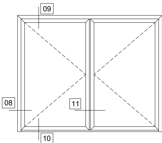
DOUBLE LEAF ENTRANCE DOOR OPENING OUTWARD ΔΙΦΥΛΛΗ ΠΟΡΤΑ ΕΙΣΟΔΟΥ ΑΝΟΙΓΟΜΕΝΗ ΕΞΩ
