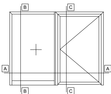
SINGLE LEAF DOOR INWARD OPENING WITH GLASS PANEL, WITHOUT THRESHOLD AND ONE FIXED SIDE PANEL WITH KICKPLATE ΜΟΝΟΦΥΛΛΗ ΠΟΡΤΑ ΑΝΟΙΓΟΜΕΝΗ ΜΕΣΑ ΜΕ ΥΑΛΟΠΙΝΑΚΑ, ΧΩΡΙΣ ΚΑΤΩΚΑΣΙ ΚΑΙ ΕΝΑ ΣΤΑΘΕΡΟ ΜΕ ΤΑΜΠΛΑ
