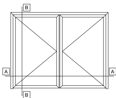
DOUBLE LEAF DOOR INWARD OPENING WITH GLASS PANEL, WITHOUT THRESHOLD ΔΙΦΥΛΛΗ ΠΟΡΤΑ ΑΝΟΙΓΟΜΕΝΗ ΜΕΣΑ ΜΕ ΥΑΛΟΠΙΝΑΚΑ, ΧΩΡΙΣ ΚΑΤΟΚΑΣΙ
