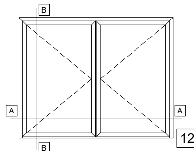
DOUBLE LEAF DOOR INWARD OPENING WITH GLASS PANEL, WITH LOW THRESHOLD ΔΙΦΥΛΛΗ ΠΟΡΤΑ ΑΝΟΙΓΟΜΕΝΗ ΜΕΣΑ ΜΕ ΥΑΛΟΠΙΝΑΚΑ, ΜΕ ΧΑΜΗΛΟ ΚΑΤΩΚΑΣΙ
