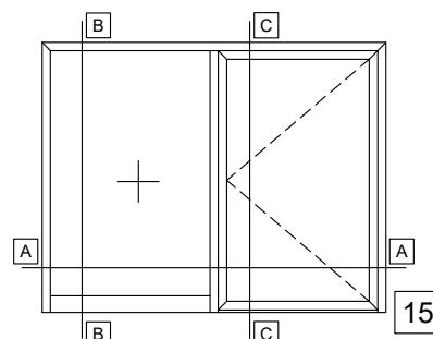
SINGLE LEAF DOOR INWARD OPENING WITH GLASS PANEL, WITH LOW THRESHOLD AND ONE FIXED SIDE PANEL WITH TRANSOM AND KICKPLATE ΜΟΝΟΦΥΛΛΗ ΠΟΡΤΑ ΑΝΟΙΓΟΜΕΝΗ ΜΕΣΑ ΜΕ ΥΑΛΟΠΙΝΑΚΑ, ΜΕ ΧΑΜΗΛΟ ΚΑΤΩΚΑΣΙ ΚΑΙ ΕΝΑ ΣΤΑΘΕΡΟ ΜΕ ΤΑΥ ΚΑΙ ΤΑΜΠΛΑ
