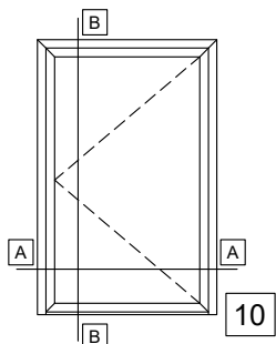
SINGLE LEAF DOOR INWARD OPENING WITH GLASS PANEL, WITH LOW THRESHOLD ΜΟΝΟΦΥΛΛΗ ΠΟΡΤΑ ΑΝΟΙΓΟΜΕΝΗ ΜΕΣΑ ΜΕ ΥΑΛΟΠΙΝΑΚΑ, ΜΕ ΧΑΜΗΛΟ ΚΑΤΩΚΑΣΙ
