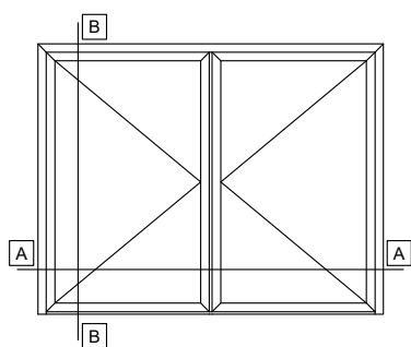
DOUBLE LEAF DOOR INWARD OPENING WITH GLASS PANEL, WITH LOW THRESHOLD ΔΙΦΥΛΛΗ ΠΟΡΤΑ ΑΝΟΙΓΟΜΕΝΗ ΜΕΣΑ ΜΕ ΥΑΛΟΠΙΝΑΚΑ, ΜΕ ΧΑΜΗΛΟ ΚΑΤΩΚΑΣΙ
