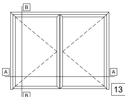
DOUBLE LEAF DOOR INWARD OPENING WITH GLASS PANEL, WITHOUT THRESHOLD ΔΙΦΥΛΛΗ ΠΟΡΤΑ ΑΝΟΙΓΟΜΕΝΗ ΜΕΣΑ ΜΕ ΥΑΛΟΠΙΝΑΚΑ, ΧΩΡΙΣ ΚΑΤΩΚΑΣΙ
