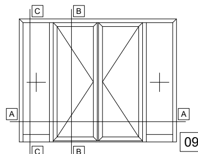
09 DOUBLE LEAF DOOR INWARD OPENING WITH GLASS PANEL, WITH TWO FIXED SIDE PANELS ΔΙΦΥΛΛΗ ΠΟΡΤΑ ΑΝΟΙΓΟΜΕΝΗ ΜΕΣΑ ΜΕ ΥΑΛΟΠΙΝΑΚΑ, ΜΕ ΔΥΟ ΣΤΑΘΕΡΑ ΕΚΑΤΕΡΩΘΕΝ
