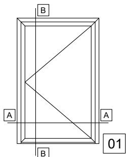
01 SINGLE LEAF DOOR INWARD OPENING WITH GLASS PANEL, WITH LOW THRESHOLD ΜΟΝΟΦΥΛΛΗ ΠΟΡΤΑ ΑΝΟΙΓΟΜΕΝΗ ΜΕΣΑ ΜΕ ΥΑΛΟΠΙΝΑΚΑ, ΜΕ ΧΑΜΗΛΟ ΚΑΤΩΚΑΣΙ
