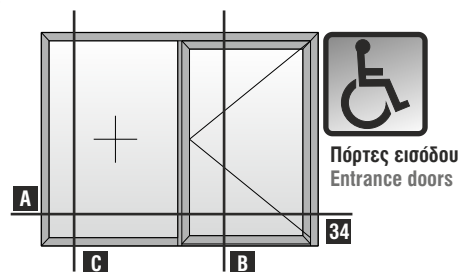
Μονόφυλλη ανοιγόμενη πόρτα με ένα σταθερό και ταμπλά- ανοιγόμενη μέσα One sash door with fixed panel and Kickplate -inwards opening
