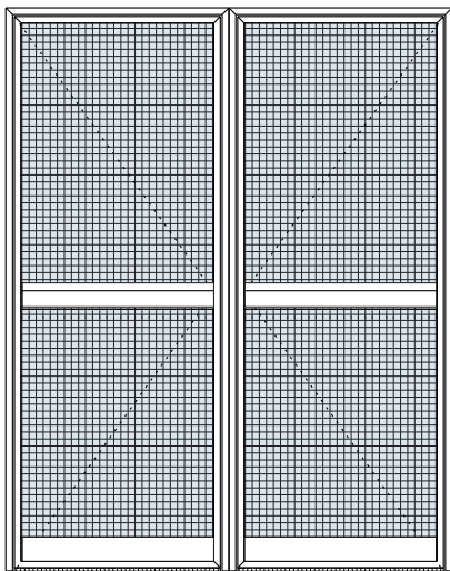
Δίφυλλη σίτα με ταμπλά Double sash insect screen with kickplate
