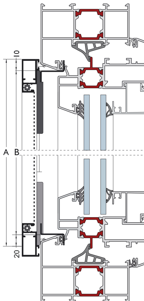
Τομή σταθερής σίτας σε ανοιγόμενο παράθυρο. Fixed fly-screen section on opening window.
