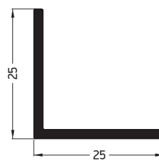
Γ-25x25x3
