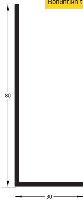
Γ-80x30x1,5
