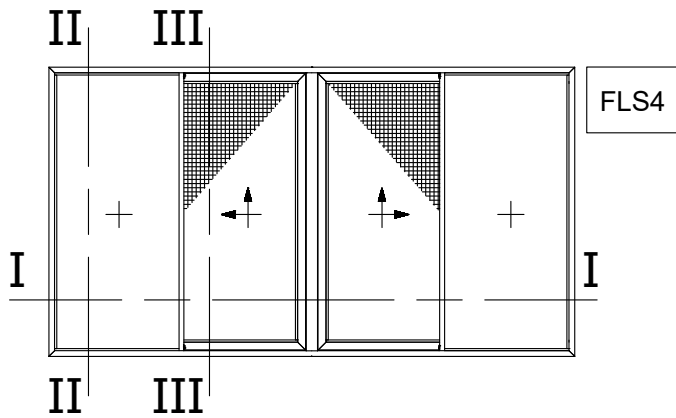
Four Sash Meeting Stile Monorail Lift and Slide with Flyscreen Τετράφυλλο Φιλητό Ανάσυρόμενο με οδηγό Monorail με Σίτα
