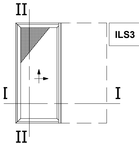
Single Sash Pocket Lift&Slide Window with Narrow Flyscreen Μονόφυλλο Χωνευτό Ανασυρόμενο με Στενή Σήτα
