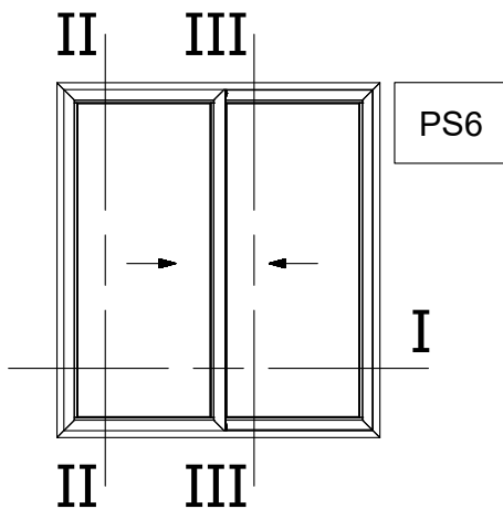
Two Sash Sliding Window 45° Cut (Sash M4542) Right Δίφυλλο Επαλλάγιο με κοπή 45° (Φύλλο M4542) Δεξιά Συρόμενο
