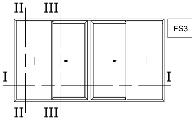
Four Sash Sliding Meeting Stile Monorail Τετράφυλλο Φιλητό Συρόμενο με οδηγό Monorail
