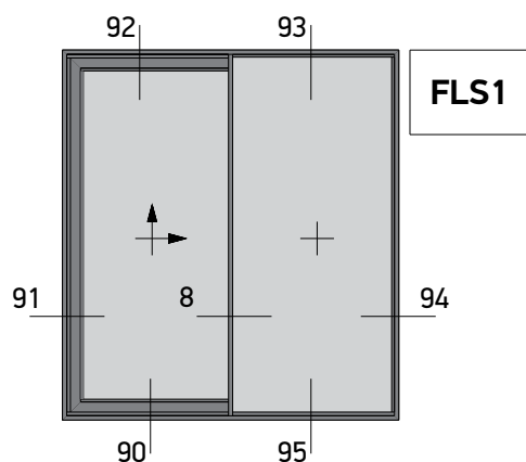
Fixed - Lift & Slide Window with Fixed on the Inside Right Σταθερό - Ανάσπυρόμενο με το Σταθερό Εσωτερικά Δεξιά Ανάσπυρόμενο
