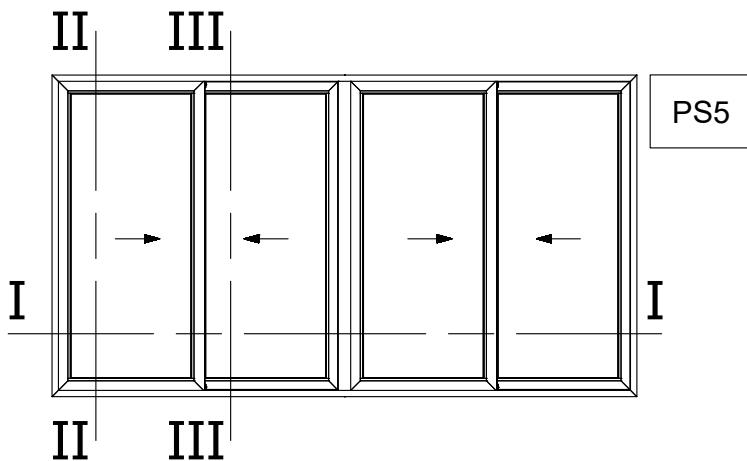
Four Sash Sliding Window 45° Cut Right Τετράφυλλο Επαλληλο με κοπή 45° Δεξιά Συρόμενο
