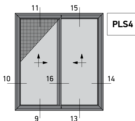
Two Sash Lift and Slide 90° Cut with Flyscreen Right Δίφυλλο Επαλλήλο με κοπή 90° και Σήτα Δεξιά Ανάστρομένο
