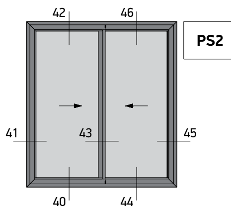
Two Sash Sliding Window 90° Cut Right Δίφυλλο Επαύλτητο με κοπή 90° Δεξιά Συρόμενο
