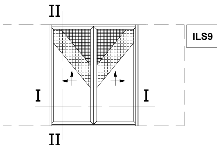
Pocket Lift&Slide Window with Meeting Stile, with Flyscreen and Shutter Χωνευτό Ανασυρόμενο Φιλητό με Σήτα και Παντζούρι
