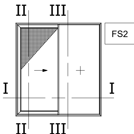
Fixed - Right Sliding Window with Fixed on the Inside and Flyscreen Σταθερό - Δεξιά Συρόμενο με το Σταθερό Εσωτερικά και Σίτα
