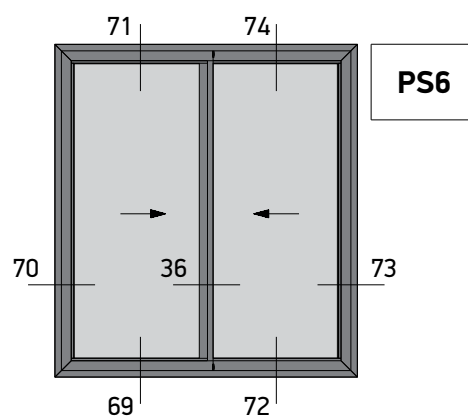
Two Sash Sliding Window 45° Cut (Sash M4542) Right Δίφυλλο Επαύλτητο με κοπή 45° (Φύλλο M4542) Δεξιά Συρόμενο
