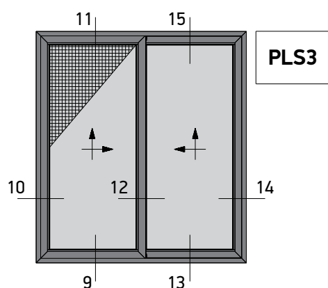
Two Sash Lift and Slide 45° Cut with Flyscreen Right Δίφυλλο Επαλλήλο με κοπή 45° και Σήτα Δεξιά Ανάστρομένο
