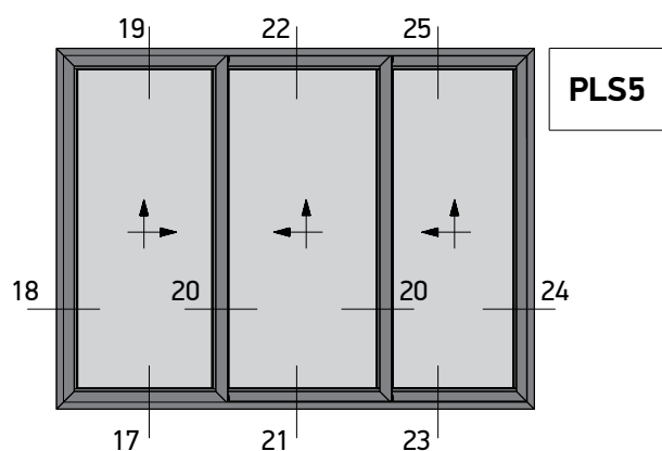
Three Sash Lift and Slide 45° Cut Right Τρίφυλλο Επαλλήλο με κοπή 45° Δεξιά Ανάστρομένο
