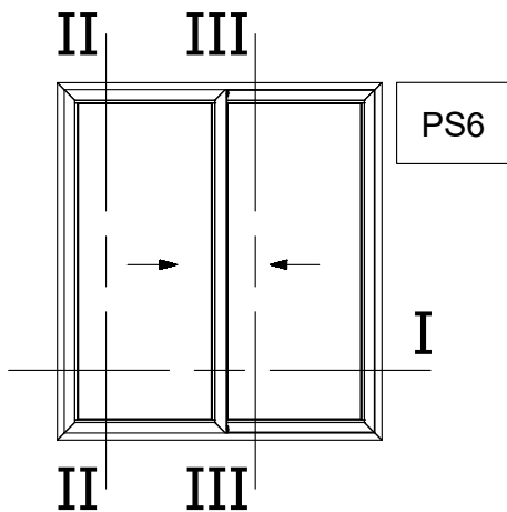
Two Sash Sliding Window 45° Cut (Sash M4542) Right Δίφυλλο Επαλλάγηλο με κοπή 45° (Φύλλο M4542) Δεξιά Συρόμενο
