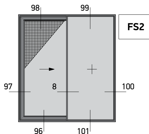
Fixed - Right Sliding Window with Fixed on the Inside and Flyscreen Σταθερό - Δεξιά Συρόμενο με το Σταθερό Εσωτερικά και Σίτα
