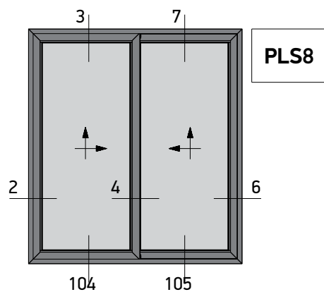
Two Sash Lift and Slide 45° Cut Right with subsill Δίφυλλο Επάλληλο με κοπή 45° Δεξιά Ανάσπυρόμενο και υδατοθεκάνη
