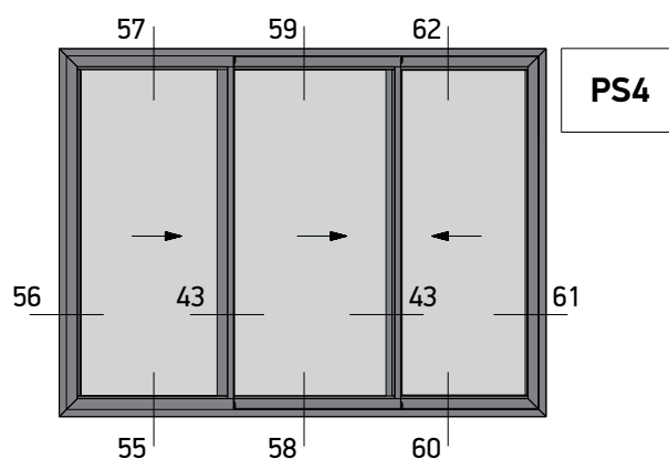
Three Sash Sliding Window 90° Cut Right Τρίφυλλο Επαύλτητο με κοπή 90° Δεξιά Συρόμενο
