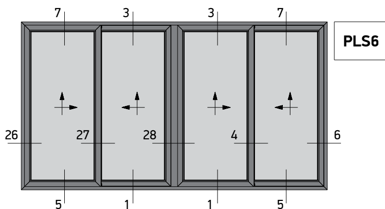
Four Sash Lift and Slide 45° Cut Right Τετράφυλλο Επάλληλο με κοπή 45° Δεξιά Ανάσπυρόμενο
