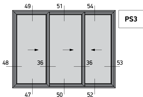
Three Sash Sliding Window 45° Cut Right Τρίφυλλο Επαύλτητο με κοπή 45° Δεξιά Συρόμενο
