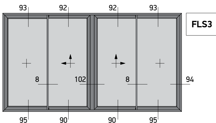
Four Sash Meeting Stile Monorail Lift and Slide Τετράφυλλο Φιλήτο Ανάσπυρόμενο με οδηγό Monorail
