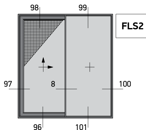
Fixed - Lift & Slide Window with Fixed on the Inside and Flyscreen Right Σταθερό - Δεξιά Ανάσπυρόμενο με το Σταθερό Εσωτερικά και Σίτα
