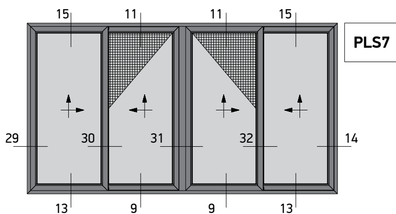
Four Sash Lift and Slide 45° Cut with Flyscreen Right Τετράφυλλο Επάλληλο με κοπή 45° και Σήτα Δεξιά Ανάσπυρόμενο
