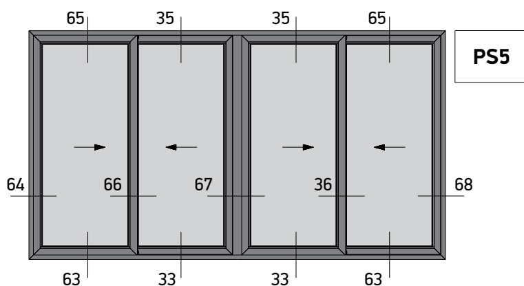
Four Sash Sliding Window 45° Cut Right Τετράφυλλο Επαύλτητο με κοπή 45° Δεξιά Συρόμενο
