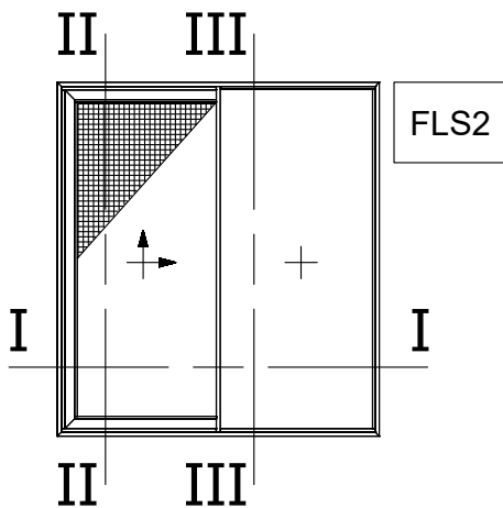
Fixed - Lift & Slide Window with Fixed on the Inside and Flyscreen Right Σταθερό - Δεξιά Ανάσυρόμενο με το Σταθερό Εσωτερικά και Σίτα
