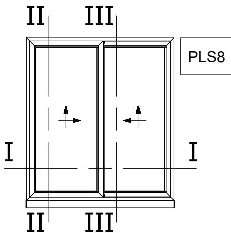
Two Sash Lift and Slide 45° Cut Right with subsill Δίφυλλο Επάλληλο με κοπή 45° Δεξιά Ανάσυρόμενο και υδατολεκάνη
