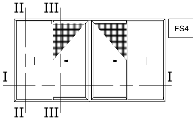
Four Sash Sliding Meeting Stile Monorail with Flyscreen Τετράφυλλο Φιλητό Συρόμενο με οδηγό Monorail με Σίτα
