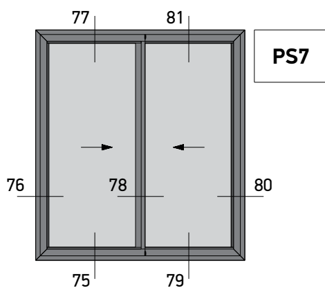
Two Sash Sliding Window 90° Cut (Sash M4544) Right Δίφυλλο Επάλληλο με κοπή 90° (Φύλλο M4544) Δεξιά Συρόμενο
