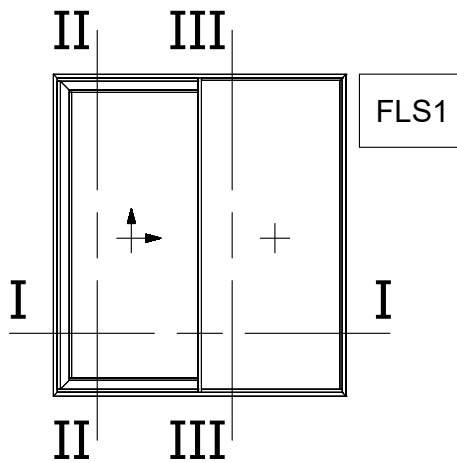
Fixed - Lift & Slide Window with Fixed on the Inside Right Σταθερό - Ανάσυρόμενο με το Σταθερό Εσωτερικά Δεξιά Ανασυρόμενο
