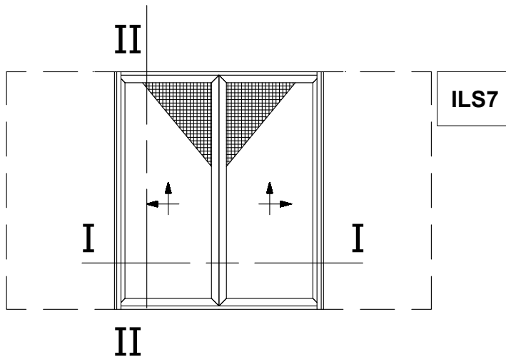
Pocket Lift&Slide Window with Meeting Stile and Flyscreen Χωνευτό Ανασπρόμενο Φιλητό με Σήτα
