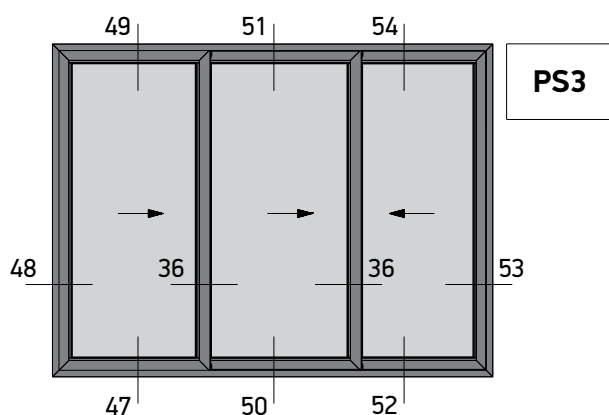
Three Sash Sliding Window 45° Cut Right Τρίφυλλο Επάλληλο με κοπή 45° Δεξιά Συρόμενο
