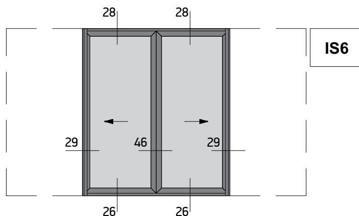
Pocket Sliding Window with Meeting Stile Χωνευτό Συρόμενο Φιλήντο
