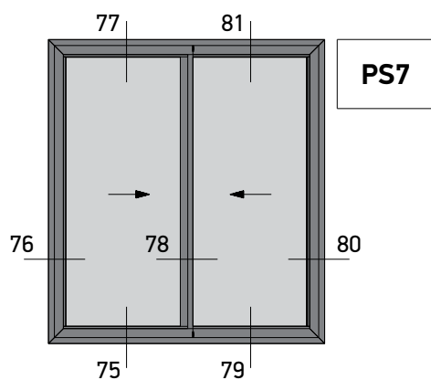
Two Sash Sliding Window 90° Cut (Sash M4544) Right Δίφυλλο Επάλληλο με κοπή 90° (Φύλλο M4544) Δεξιά Συρόμενο
