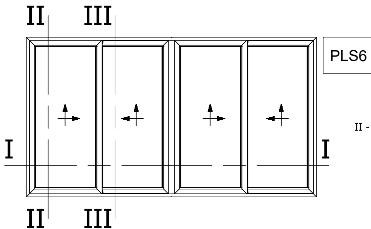
Four Sash Lift and Slide 45° Cut Right Τετράφυλλο Επάλληλο με κοπή 45° Δεξιά Ανάσυρόμενο
