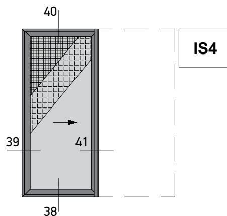
Single Sash Pocket Sliding Window with Flyscreen and Shutter Μονόφυλλο Χωνευτό Συρόμενο με Σήτα και Παντζούρι
