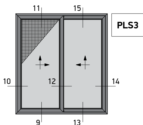
Two Sash Lift and Slide 45° Cut with Flyscreen Right Δίφυλλο Επαλλήλο με κοπή 45° και Σήτα Δεξιά Ανάσυρόμενο
