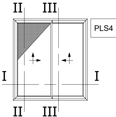
Two Sash Lift and Slide 90° Cut with Flyscreen Right Δίφυλλο Επαλληλο με κοπή 90° και Σήτα Δεξιά Ανάσυρόμενο
