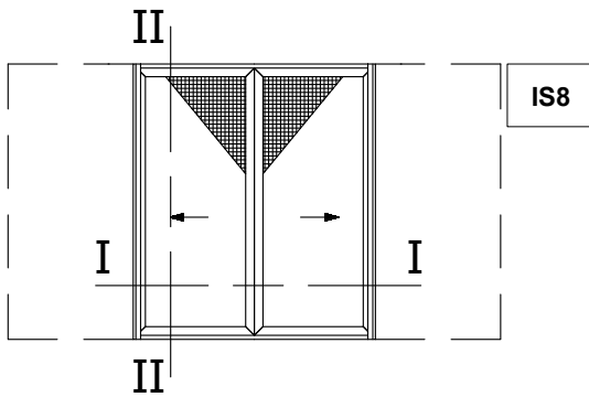
Pocket Sliding Window with Meeting Stile and Narrow Flyscreen Χωνευτό Συρόμενο Φιλητό με Στενή Σήτα
