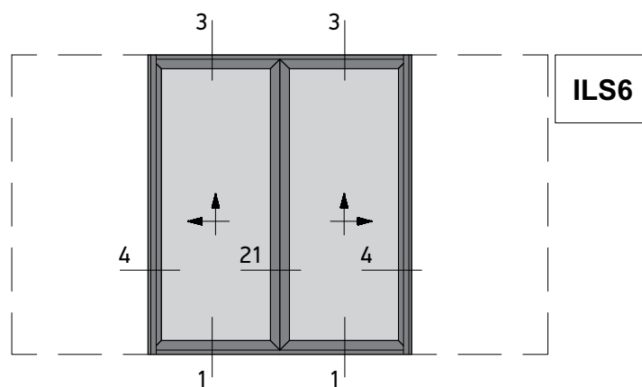
Pocket Lift&Slide Window with Meeting Stile Χωνευτό Ανασπώμενο Φιλητό
