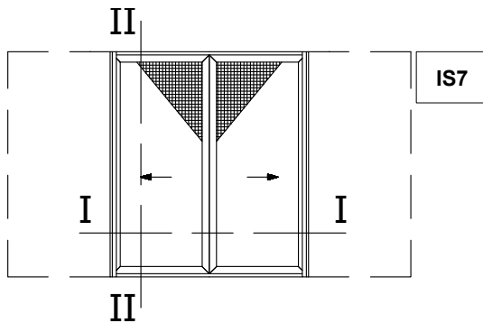
Pocket Sliding Window with Meeting Stile and Flyscreen Χωνευτό Συρόμενο Φιλητό με Σήτα
