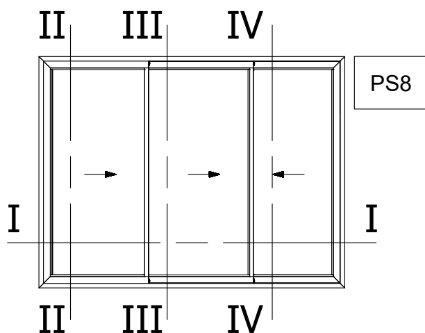
Three Sash Sliding Window 90° Cut (Sash M4544) Right Τρίφυλλο Επάλληλο με κοπή 90° (φύλλο M4544) Δεξιά Συρόμενο
