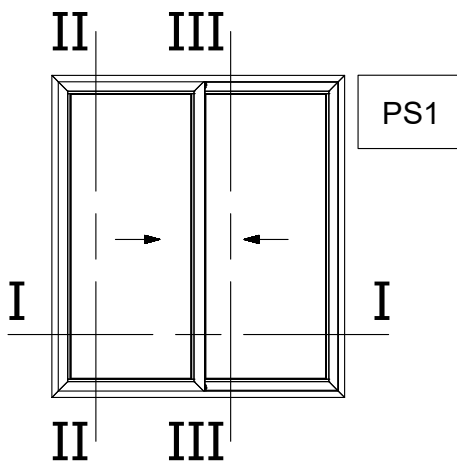
Two Sash Sliding Window 45° Cut Right Δίφυλλο Επαλλάγιο με κοπή 45° Δεξιά Συρόμενο
