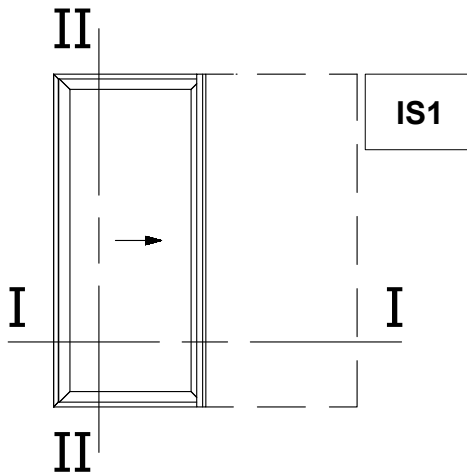
Single Sash Pocket Sliding Window Μονόφυλλο Χωνευτό Συρόμενο
