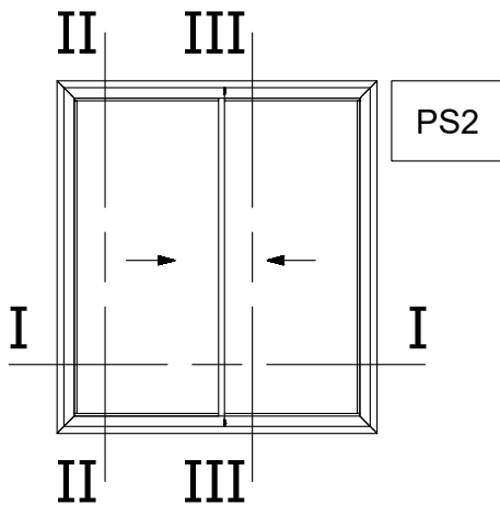
Two Sash Sliding Window 90° Cut Right Δίφυλλο Επάλληλο με κοπή 90° Δεξιά Συρόμενο
