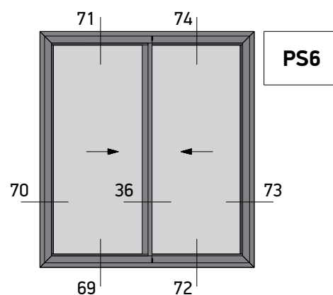
Two Sash Sliding Window 45° Cut (Sash M4542) Right Δίφυλλο Επάλληλο με κοπή 45° (Φύλλο M4542) Δεξιά Συρόμενο
