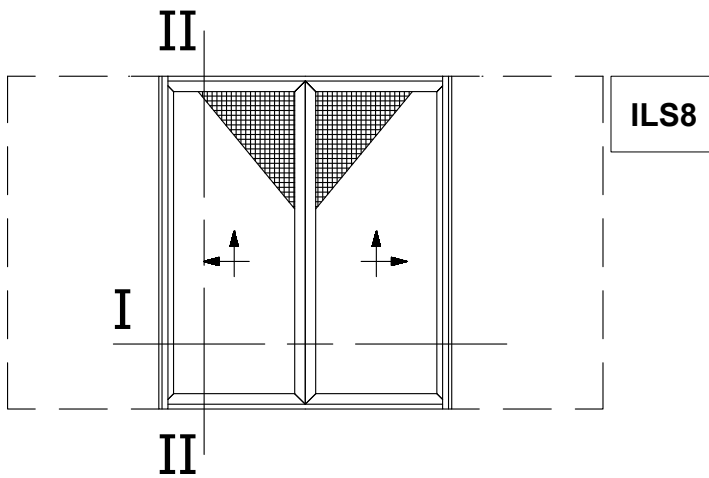
Pocket Lift&Slide Window with Meeting Stile and Narrow Flyscreen Χωνευτό Ανασυρόμενο Φιλητό με Στενή Σήτα
