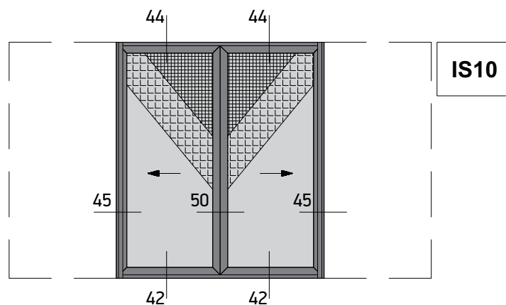
Pocket Sliding Window with Meeting Stile, with Narrow Flyscreen and Shutter Χωνευτό Συρόμενο Φιλιπτό με Στενή Σήτα και Παντζούρι
