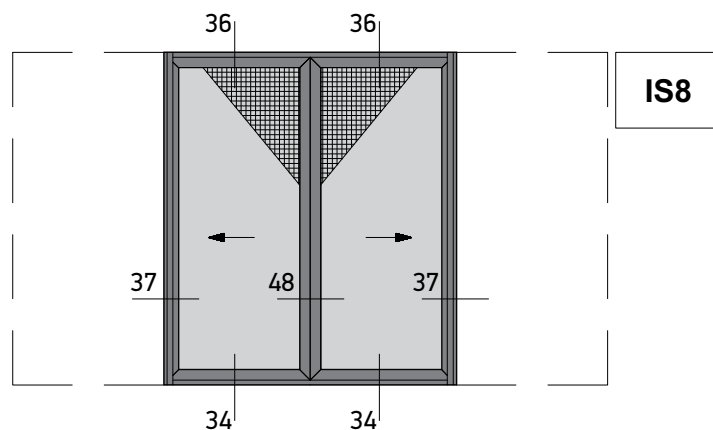
Pocket Sliding Window with Meeting Stile and Narrow Flyscreen Χωνευτό Συρόμενο Φιλιπτό με Στενή Σήτα
