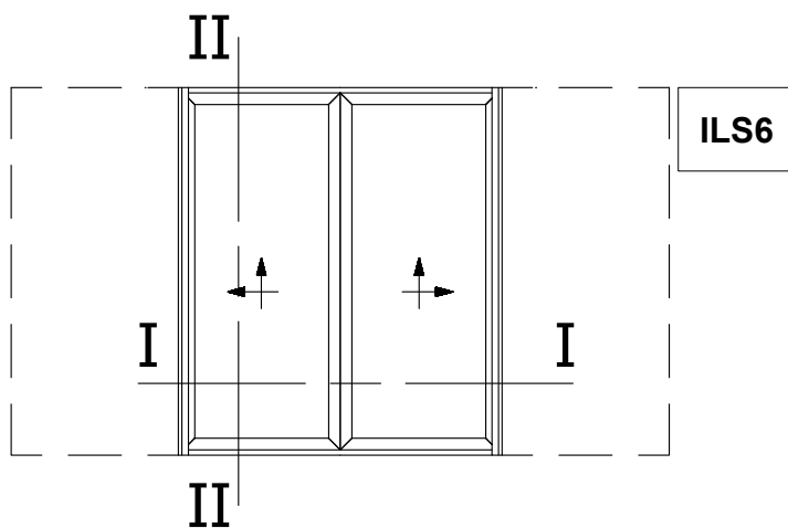
Pocket Lift&Slide Window with Meeting Stile Χωνευτό Ανασυρόμενο Φιλητό
