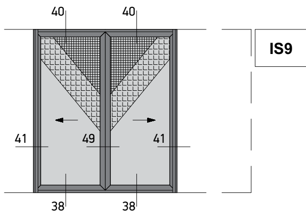
Pocket Sliding Window with Meeting Stile, with Flyscreen and Shutter Χωνευτό Συρόμενο Φιλιπτό με Σήτα και Παντζούρι
