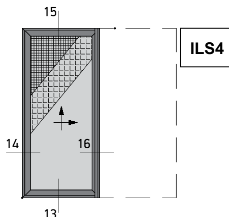
Single Sash Pocket Lift&Slide Window with Flyscreen and Shutter Μονόφυλλο Χωνευτό Ανασπώμενο με Σήτα και Παντζούρι
