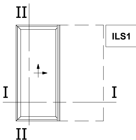
Μονόφυλλο Χωνευτό Ανασυρόμενο Single Sash Pocket Lift&Slide Window
