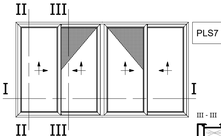
Four Sash Lift and Slide 45° Cut with Flyscreen Right Τετράφυλλο Επάλληλο με κοπή 45° και Σήτα Δεξιά Ανάσυρόμενο
