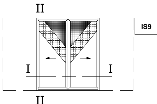
Pocket Sliding Window with Meeting Stile, with Flyscreen and Shutter Χωνευτό Συρόμενο Φιλητό με Σήτα και Παντζούρι
