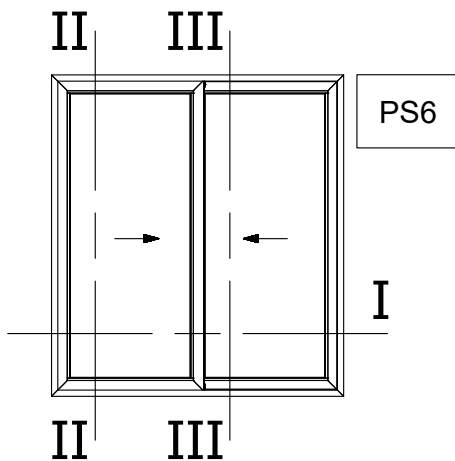
Two Sash Sliding Window 45° Cut (Sash M4542) Right Δίφυλλο Επάλληλο με κοπή 45° (Φύλλο M4542) Δεξιά Συρόμενο
