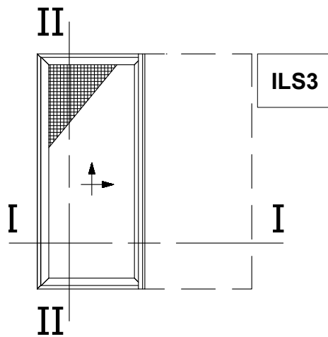
Single Sash Pocket Lift&Slide Window with Narrow Flyscreen Μονόφυλλο Χωνευτό Ανασυρόμενο με Στενή Σήτα
