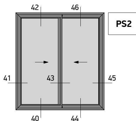
Two Sash Sliding Window 90° Cut Right Δίφυλλο Επάλληλο με κοπή 90° Δεξιά Συρόμενο
