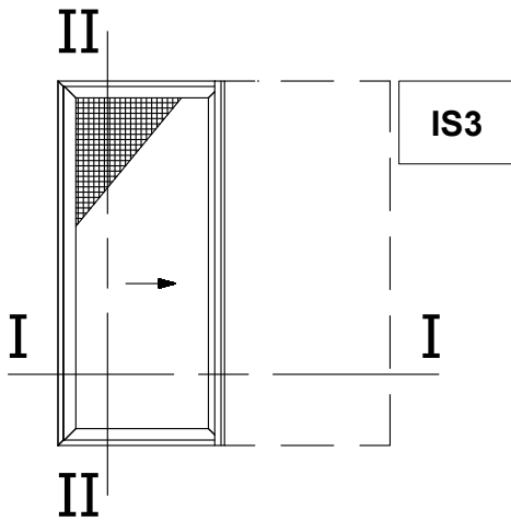
Single Sash Pocket Sliding Window with Narrow Flyscreen Μονόφυλλο Χωνευτό Συρόμενο με Στενή Σήτα
