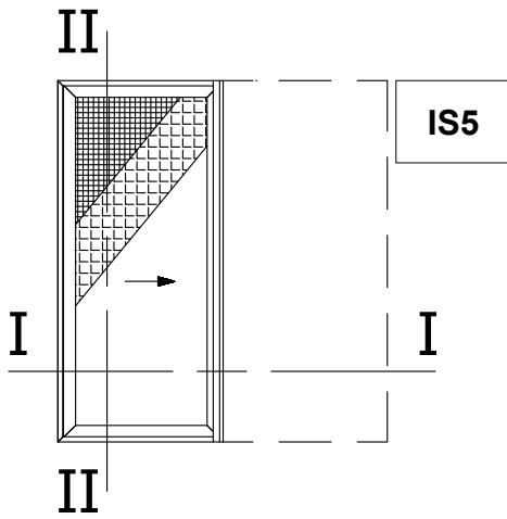
Single Sash Pocket Sliding Window with Narrow Flyscreen and Shutter Μονόφυλλο Χωνευτό Συρόμενο με Στενή Σήτα και Παντζούρι
