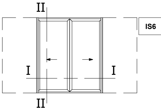
Pocket Sliding Window with Meeting Stile Χωνευτό Συρόμενο Φιλητό
