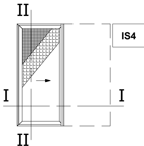
Single Sash Pocket Sliding Window with Flyscreen and Shutter Μονόφυλλο Χωνευτό Συρόμενο με Σήτα και Παντζούρι
