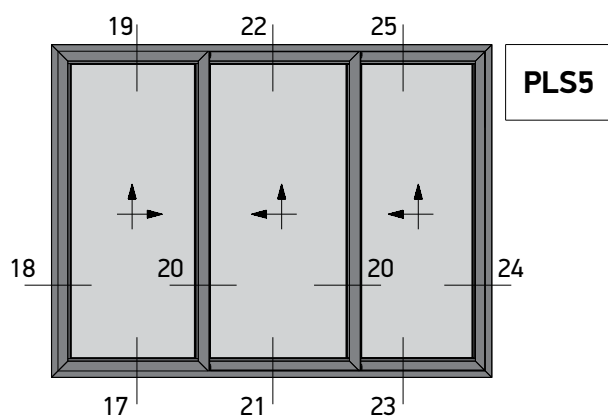
Three Sash Lift and Slide 45° Cut Right Τρίφυλλο Επαλλήλο με κοπή 45° Δεξιά Ανάσυρόμενο
