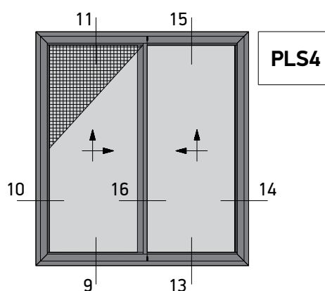
Two Sash Lift and Slide 90° Cut with Flyscreen Right Δίφυλλο Επαλλήλο με κοπή 90° και Σήτα Δεξιά Ανάσυρόμενο
