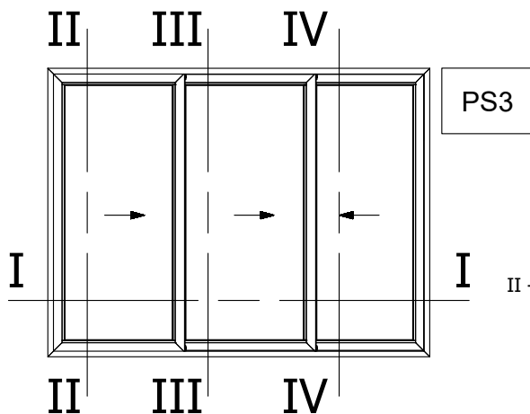
Three Sash Sliding Window 45° Cut Right Τρίφυλλο Επάλληλο με κοπή 45° Δεξιά Συρόμενο
