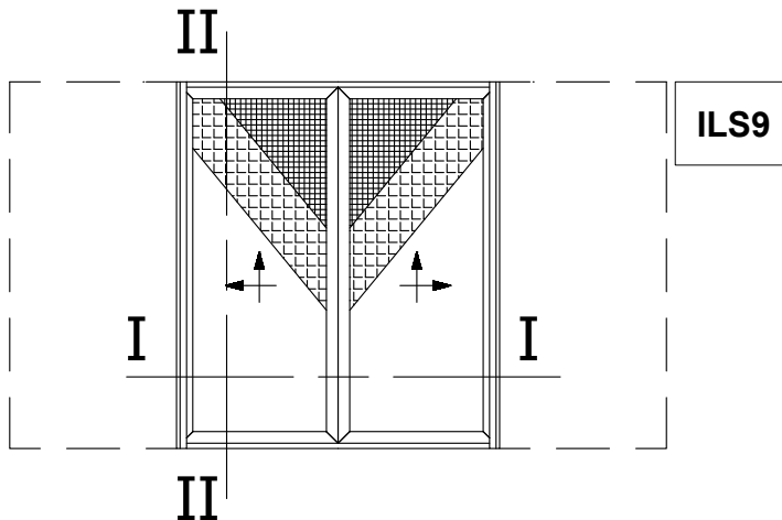
Pocket Lift&Slide Window with Meeting Stile, with Flyscreen and Shutter Χωνευτό Ανασπρόμενο Φιλητό με Σήτα και Παντζούρι
