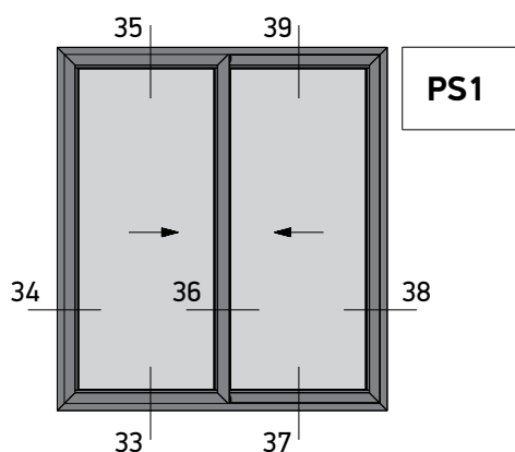
Two Sash Sliding Window 45° Cut Right Δίφυλλο Επάλληλο με κοπή 45° Δεξιά Συρόμενο
