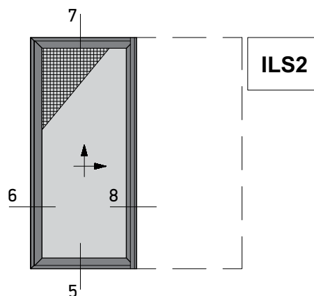
Single Sash Pocket Lift&Slide Window with Flyscreen Μονόφυλλο Χωνευτό Ανασπώμενο με Σήτα
