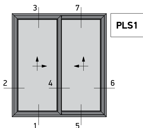
Two Sash Lift and Slide 45° Cut Right Δίφυλλο Επαλλήλο με κοπή 45° Δεξιά Ανάσυρόμενο
