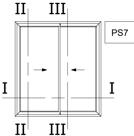
Two Sash Sliding Window 90° Cut (Sash M4544) Right Δίφυλλο Επτάλληλο με κοπή 90° (Φύλλο M4544) Δεξιά Συρόμενο
