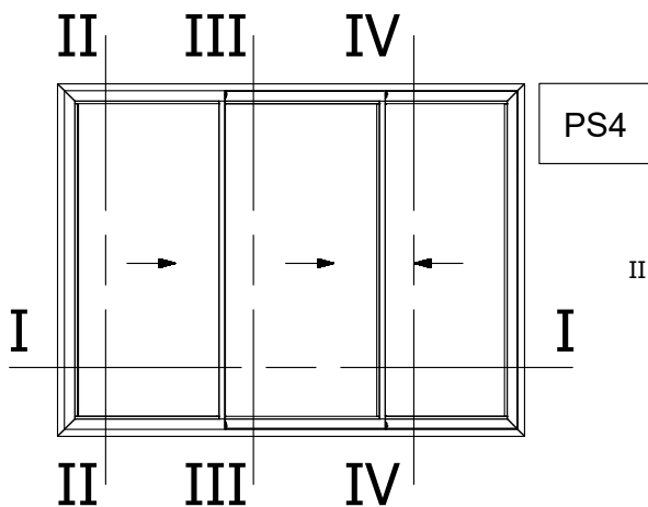
Three Sash Sliding Window 90° Cut Right Τρίφυλλο Επάλληλο με κοπή 90° Δεξιά Συρόμενο
