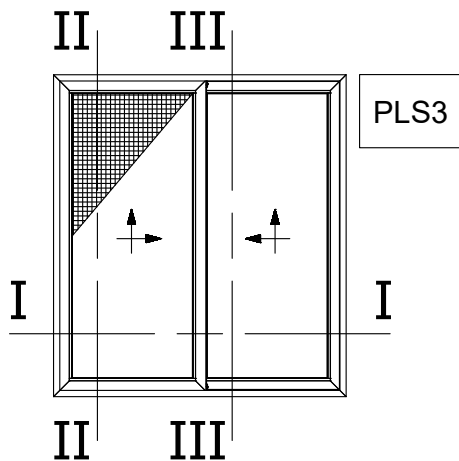
Two Sash Lift and Slide 45° Cut with Flyscreen Right Δίφυλλο Επάλληλο με κοπή 45° και Σήτα Δεξιά Ανάσυρόμενο
