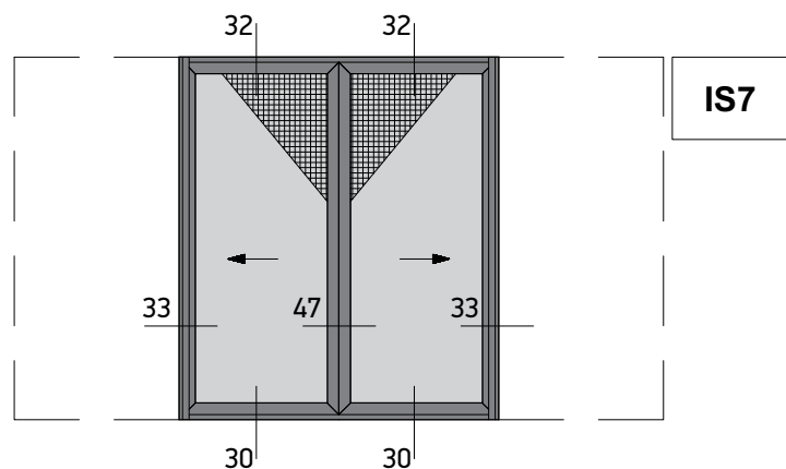
Pocket Sliding Window with Meeting Stile and Flyscreen Χωνευτό Συρόμενο Φιλιπτό με Σήτα
