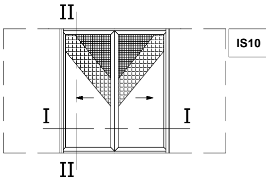
Pocket Sliding Window with Meeting Stile, with Narrow Flyscreen and Shutter Χωνευτό Συρόμενο Φιλητό με Στενή Σήτα και Παντζούρι
