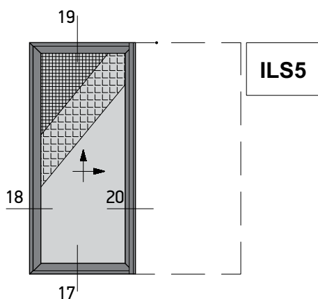
Single Sash Pocket Lift&Slide Window with Narrow Flyscreen and Shutter Μονόφυλλο Χωνευτό Ανασπώμενο με Στενή Σήτα και Παντζούρι
