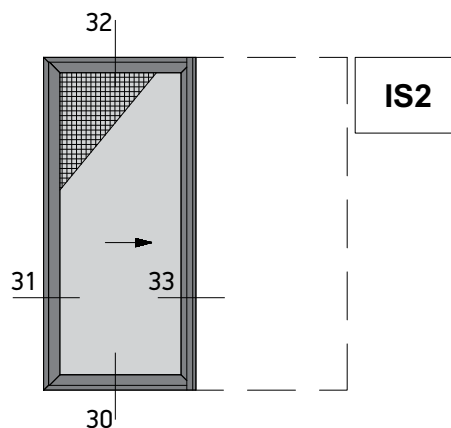
Single Sash Pocket Sliding Window with Flyscreen Μονόφυλλο Χωνευτό Συρόμενο με Σήτα
