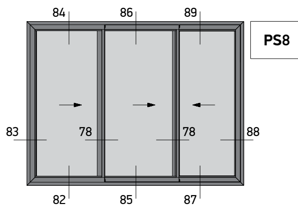
Three Sash Sliding Window 90° Cut (Sash M4544) Right Τρίφυλλο Επάλληλο με κοπή 90° (φύλλο M4544) Δεξιά Συρόμενο
