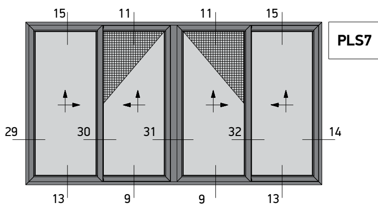
Four Sash Lift and Slide 45° Cut with Flyscreen Right Τετράφυλλο Επάλληλο με κοπή 45° και Σήτα Δεξιά Ανάσπρόμενο
