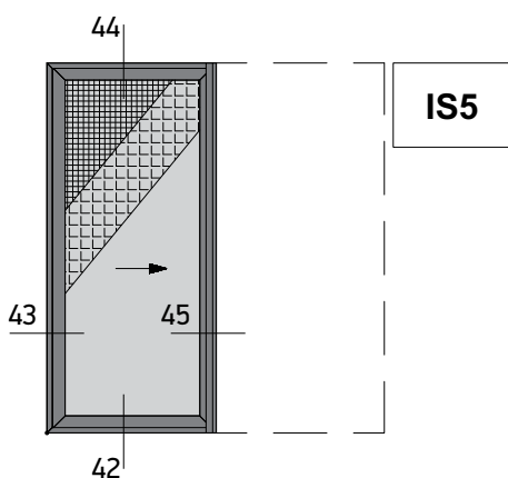
Single Sash Pocket Sliding Window with Narrow Flyscreen and Shutter Μονόφυλλο Χωνευτό Συρόμενο με Στενή Σήτα και Παντζούρι
