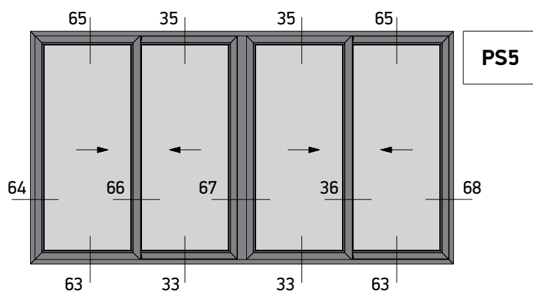
Four Sash Sliding Window 45° Cut Right Τετράφυλλο Επάλληλο με κοπή 45° Δεξιά Συρόμενο
