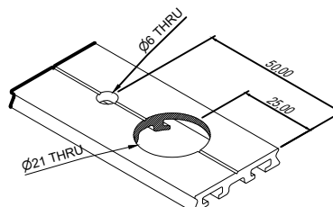
Pressure Plate Machining/ Κατεργασία Πλάκας Πίεσης
