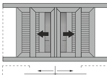
Double sash pocket sliding window in meeting stile, in 90° assembly with glass - fly screens & shutters Δίφυλλο χωνευτό με 90°/45° κοπή στο κάτω/πάνω μέρος του φύλλου, με σήτα και παντζούρι
