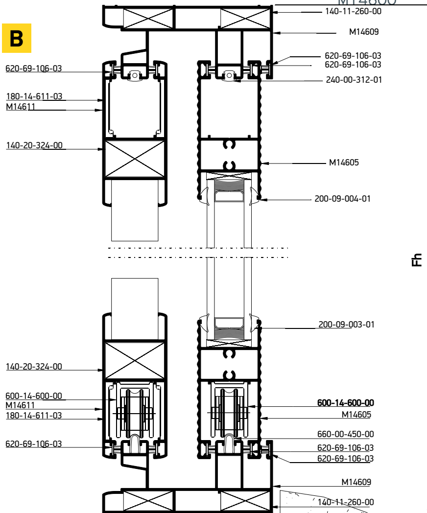
One-sash sash pocket sliding window 90° cut with shutter Μονόφυλλο χωνευτό με 90° κοπή, με παντζούρι
