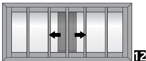
Six sash narrow parallel sliding in 90 assembly window in meeting stile with fly screen Εξάφυλλο Ενόθητο Φυλήτο 90°Κοπή, με σήτα
