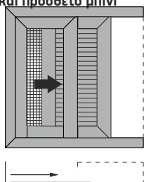
Single sash pocket sliding window in 90° assembly with glass, fly screen & shutter Μονόφυλλο χωνευτό με 90°/45° κοπή στο κάτω/πάνω μέρος του φύλλου, με σήτα και παντζούρι
