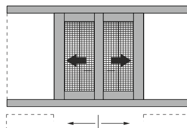
Double narrow sash pocket sliding in 90° assembly window in meeting stile with fly screen Δίφυλλο χωνευτό με 90° κοπή, με σήτα
