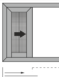
Single sash pocket sliding window in 90° assembly with fly screen Μονόφυλλο χωνευτό με 90°/45° κοπή στο κάτω/πάνω μέρος του φύλλου, με σήτα
