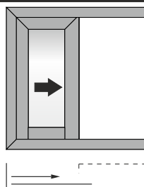
Single sash pocket sliding window in 90° assembly Μονόφυλλο χωνευτό με 90°/45° κοπή στο κάτω/πάνω μέρος του φύλλου
