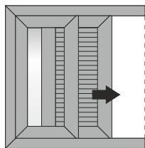
Single sash pocket sliding window with shutter Μονόφυλλο χωνευτό συρόμενο 45° κοπή με παντζούρι
