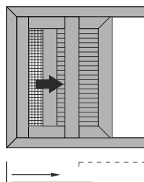
One-sash pocket sliding window 90° cut with flyscreen & shutter Μονόφυλλο χωνευτό με 90° κοπή, με σήτα και παντζούρι
