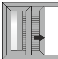
Single sash pocket sliding window in 90° assembly with shutter Μονόφυλλο χωνευτό με 90°/45° κοπή στο κάτω/πάνω μέρος του φύλλου, με παντζούρι
