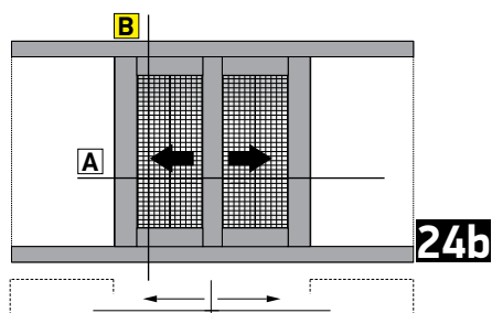
Double sash pocket sliding window 90° cut with narrow meeting stile, with flyscreen Δίφυλλο χωνευτό με 90° κοπή και στενό μπινί, με σήτα
