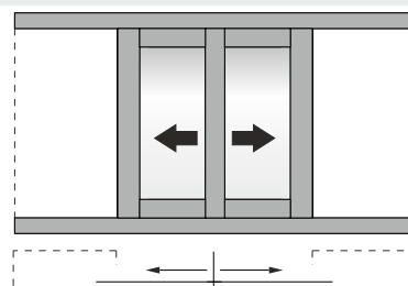
Double sash pocket sliding window 90° cut with additional meeting stile Δίφυλλο χωνευτό με 90° κοπή και πρόσθετο μπινί
