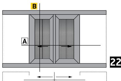
Double sash pocket sliding window in meeting stile with fly screen Δίφυλλο χωνευτό συρόμενο 45° κοπή, με σήτα
