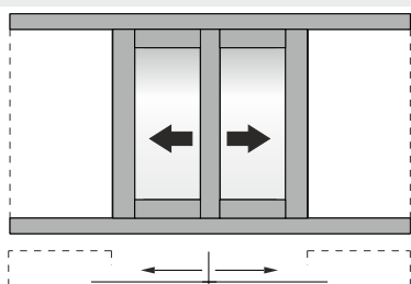
Double sash pocket sliding window 90° cut with narrow meeting stile Δίφυλλο χωνευτό με 90° κοπή και στενό μπινί
