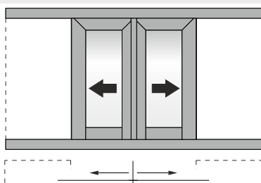
Double sash pocket sliding window assembly 90°/45° in meeting stile Δίφυλλο χωνευτό με 90°/45° κοπή στο κάτω/πάνω μέρος του φύλλου
