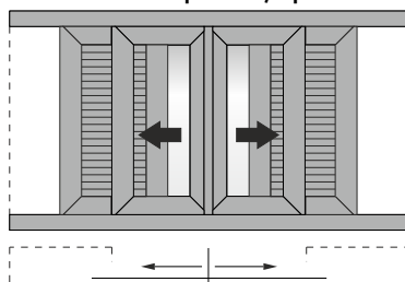
Double sash pocket sliding window in meeting stile with shutters Δίφυλλο χωνευτό συρόμενο 45° κοπή, με παντζούρι
