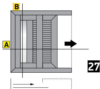
One-sash sash pocket sliding window 90° cut with shutter Μονόφυλλο χωνευτό με 90° κοπή, με παντζούρι
