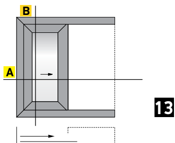
Single sash pocket sliding window Μονόφυλλο χωνευτό συρόμενο 45° κοπή
