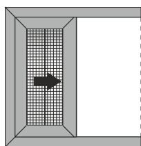
Single sash pocket sliding window with fly screen Μονόφυλλο χωνευτό συρόμενο 45° κοπή, με σήτα
