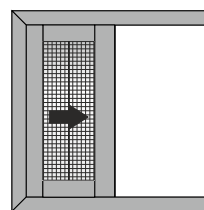
Single sash pocket sliding window in 90° assembly with fly screen Μονόφυλλο χωνευτό με 90° κοπή, με σήτα
