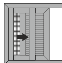
One-sash pocket sliding window 90° cut with glass, fly screen & shutter Μονόφυλλο χωνευτό με 90° κοπή, με σήτα και παντζούρι
