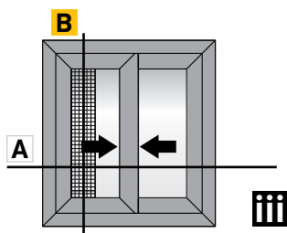
Double sliding window with flat frame & narrow flyscreen, 45° cut Δίφυλλο επάλληλο συρόμενο με χαμηλό οδογό & στενή σίτα, 45° κοπή
