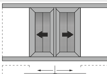
Double sash pocket sliding window in meeting stile with fly screen Δίφυλλο χωνευτό συρόμενο 45° κοπή, με σήτα
