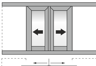
Double sash pocket sliding in 90°/45° assembly window in meeting stile Δίφυλλο χωνευτό με 90°/45° κοπή στο κάτω/πάνω μέρος του φύλλου
