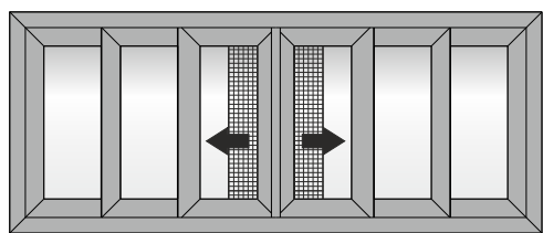
Six sash n parallel sliding window in meeting stile with fly screen Εξάφυλλο Επάλληλο 45° Κοπή, με σήτα
