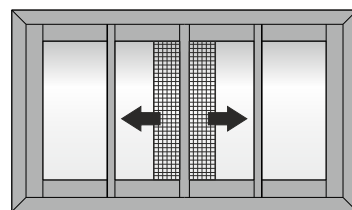
Four sash narrow parallel sliding in 90 assembly window in meeting stile with fly screen Τετράφυλλο Επάλληλο Φιλιττό 90° Κοπή, με σήτα
