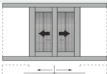
Double sash pocket sliding window 90° cut with additional meeting stile, with flyscreen Δίφυλλο χωνευτό με 90° κοπή και πρόσθετο μπινί, με σήτα
