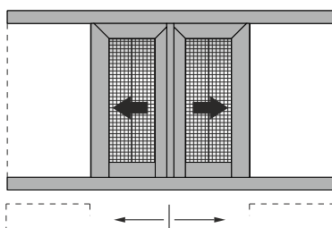
Double sash pocket sliding in 90°/45° assembly window in meeting stile with fly screen Δίφυλλο χωνευτό με 90°/45° κοπή στο κάτω/πάνω μέρος του φύλλου, με σήτα
