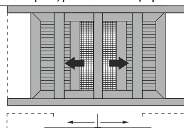
Double sash pocket sliding window in meeting stile, in 90° assembly with glass - fly screens & shutters Δίφυλλο χωνευτό με 90° κοπή, με σήτα και παντζούρι
