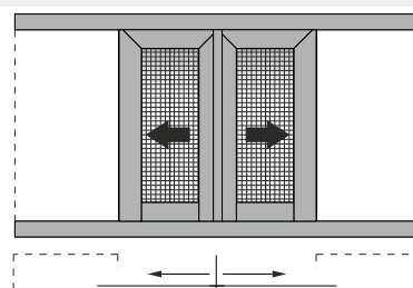
Double sash pocket sliding window in 90° assembly with fly screen Δίφυλλο χωνευτό με 90°/45° κοπή στο κάτω/πάνω μέρος του φύλλου, με σήτα
