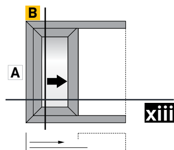
Single wall sash sliding window with flat frame, 45° cut Μονόφυλλο χωνευτό συρόμενο με χαμηλό οδηγό, 45° κοπή
