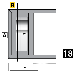
Single sash pocket sliding window in 90° assembly with fly screen Μονόφυλλο χωνευτό με 90° κοπή, με σήτα
