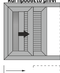
Single sash pocket sliding window with glass - fly screen & shutter Μονόφυλλο χωνευτό συρόμενο 45° κοπή,
