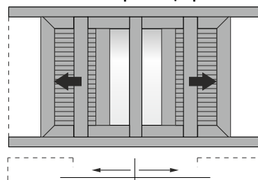
Double sash pocket sliding window with shutter 90° cut with additional meeting stile Δίφυλλο χωνευτό με 90° κοπή και πρόσθετο μπινί
