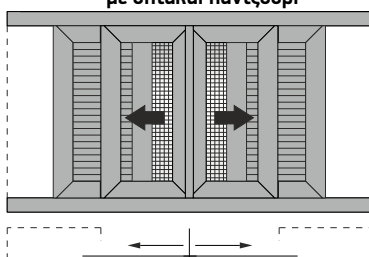
Double sash pocket sliding window in meeting stile, with glass - fly screens & shutters Δίφυλλο χωνευτό συρόμενο 45° κοπή, με σήτα και παντζούρι
