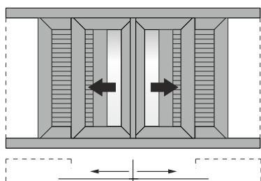
Double sash pocket sliding window 90° in meeting stile with shutters Δίφυλλο χωνευτό συρόμενο 45° κοπή, με παντζούρι
