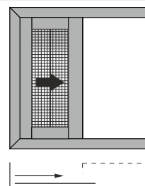
Single sash pocket sliding window in 90° assembly with fly screen Μονόφυλλο χωνευτό με 90° κοπή, με σήτα
