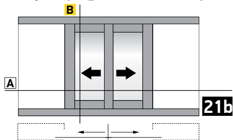
Double sash pocket sliding window 90° cut with narrow meeting stile Δίφυλλο χωνευτό με 90° κοπή και στενό μπινί
