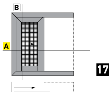
Single sash pocket sliding window in 90°/45° assembly with fly screen Μονόφυλλο χωνευτό με 90°/45° κοπή στο κάτω/πάνω μέρος του φύλλου, με σήτα
