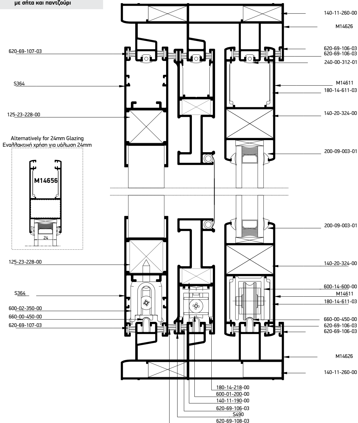
Double sash pocket sliding window in meeting stile, with glass - fly screens & shutters Δίφυλλο χωνευτό συρόμενο 45° κοπή, με σήτα και παντζούρι
