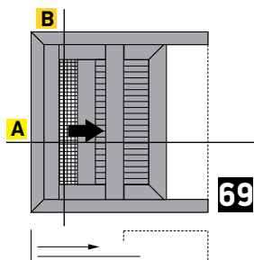
One-sash wall sliding window 90° cut with glass, fly screen & shutter Μονόφυλλο χωνευτό με 90° κοπή, με σήτα και παντζούρι
