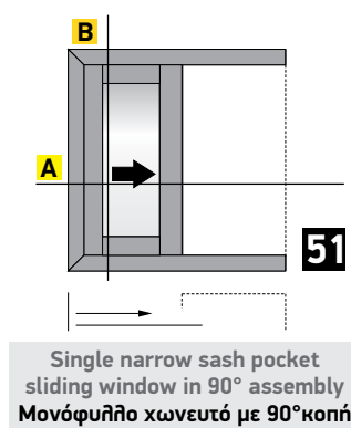
Flat frame - Χαμηλός Οδηγός
