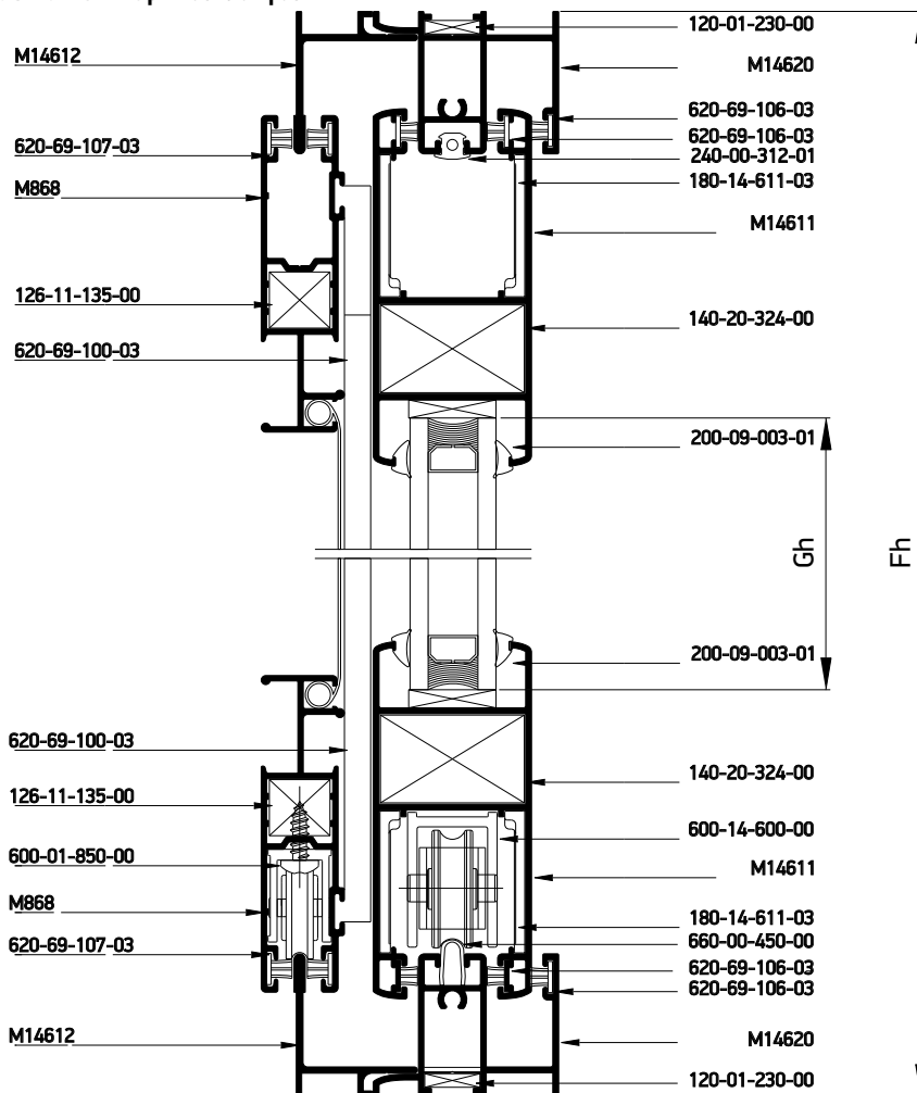
Single sash pocket sliding window with fly screen Μονόφυλλο χωνευτό συρόμενο 45° κοπή, με σήτα
