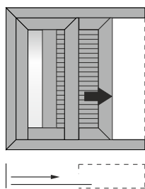
Single sash pocket sliding window in 90° assembly with shutter Μονόφυλλο χωνευτό με 90°/45° κοπή στο κάτω/πάνω μέρος του φύλλου, με παντζούρι
