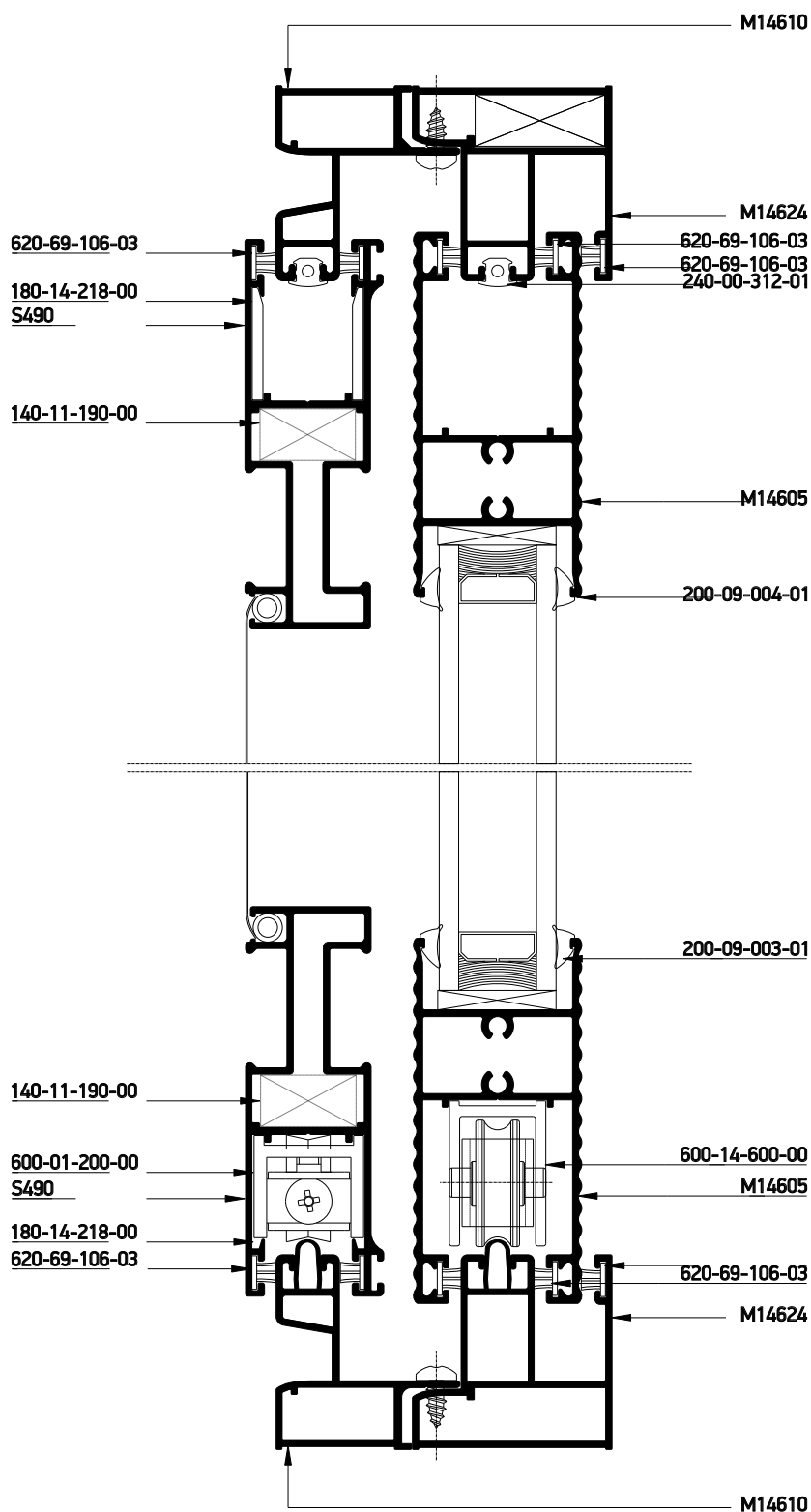
Double sash pocket sliding window 90° cut with narrow meeting stile, with flyscreen Δίφυλλο χωνευτό με 90° κοπή και στενό μπινί, με σήτα
