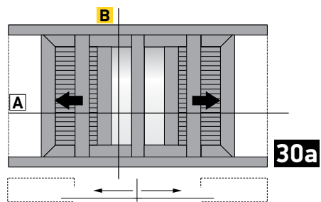
Two-sash pocket sliding window with shutter 90° cut with additional meeting stile Δίφυλλο χωνευτό με παντζούρι 90° κοπή και πρόσθετο μινί
