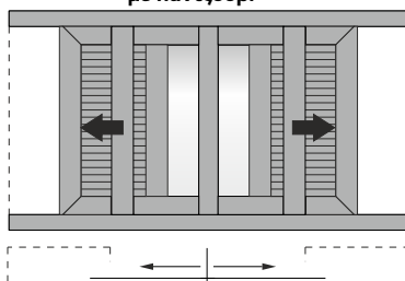
Two-sash pocket sliding window with shutter 90° cut Δίφυλλο χωνευτό με παντζούρι 90° κοπή
