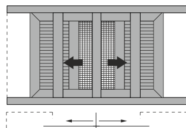
Double narrow sash pocket sliding window in meeting stile, in 90° assembly with glass - fly screens & shutters Δίφυλλο χωνευτό με 90° κοπή, με σήτα και παντζούρι
