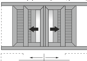
Double sash pocket sliding window in 90° assembly with shutters Δίφυλλο χωνευτό με 90°/45° κοπή στο κάτω/πάνω μέρος του φύλλου, με παντζούρι
