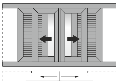
Double sash pocket sliding in 90° assembly window in meeting stile with shutters Δίφυλλο χωνευτό με 90°/45° κοπή στο κάτω/πάνω μέρος του φύλλου, με παντζούρι
