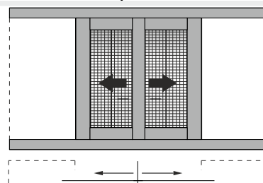
Double sash pocket sliding window 90° cut with narrow meeting stile, with flyscreen Δίφυλλο χωνευτό με 90° κοπή και στενό μπινί, με σήτα
