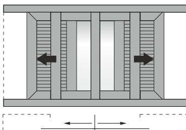
Two-sash pocket sliding window with shutter 90° cut with additional meeting stile Δίφυλλο χωνευτό με παντζούρι 90° κοπή και πρόσθετο μπινί
