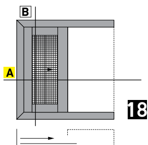
Single sash pocket sliding window in 90° assembly with fly screen Μονόφυλλο χωνευτό με 90° κοπή, με σήτα
