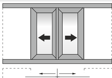
Double sash pocket sliding window in meeting stile Δίφυλλο χωνευτό συρόμενο 45° κοπή
