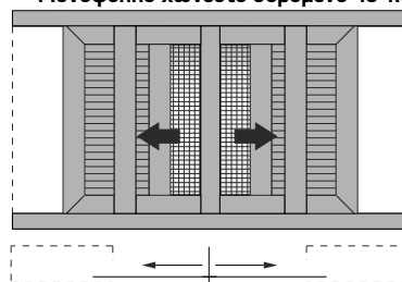
Double narrow sash pocket sliding window in meeting stile, narrow intelocking profile in 90° assembly with glass - fly screens & shutters Δίφυλλο χωνευτό με 90° κοπή, στενό μπινί, με σήτα και παντζούρι
