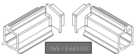
765-13-622-03 Τάπα για κατωκάσι 303022 End cap for slat 303022
