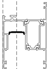
Sash S560 | Φύλλο S560
