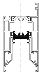
Sash M4542 | Φύλλο M4542
