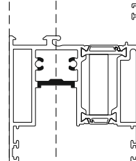
Sash S70710 | Φύλλο S70710
