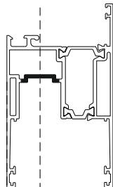
Sash S584 | Φύλλο S584
