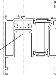
Sash S70706 | Φύλλο S70706
