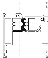
Sash S70776 | Φύλλο S70776
